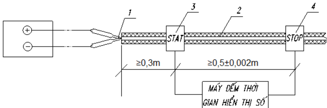
Hình 1: Sơ đồ nguyên lý xác định tốc độ truyền sóng nổ của dây dẫn tín hiệu nổ
