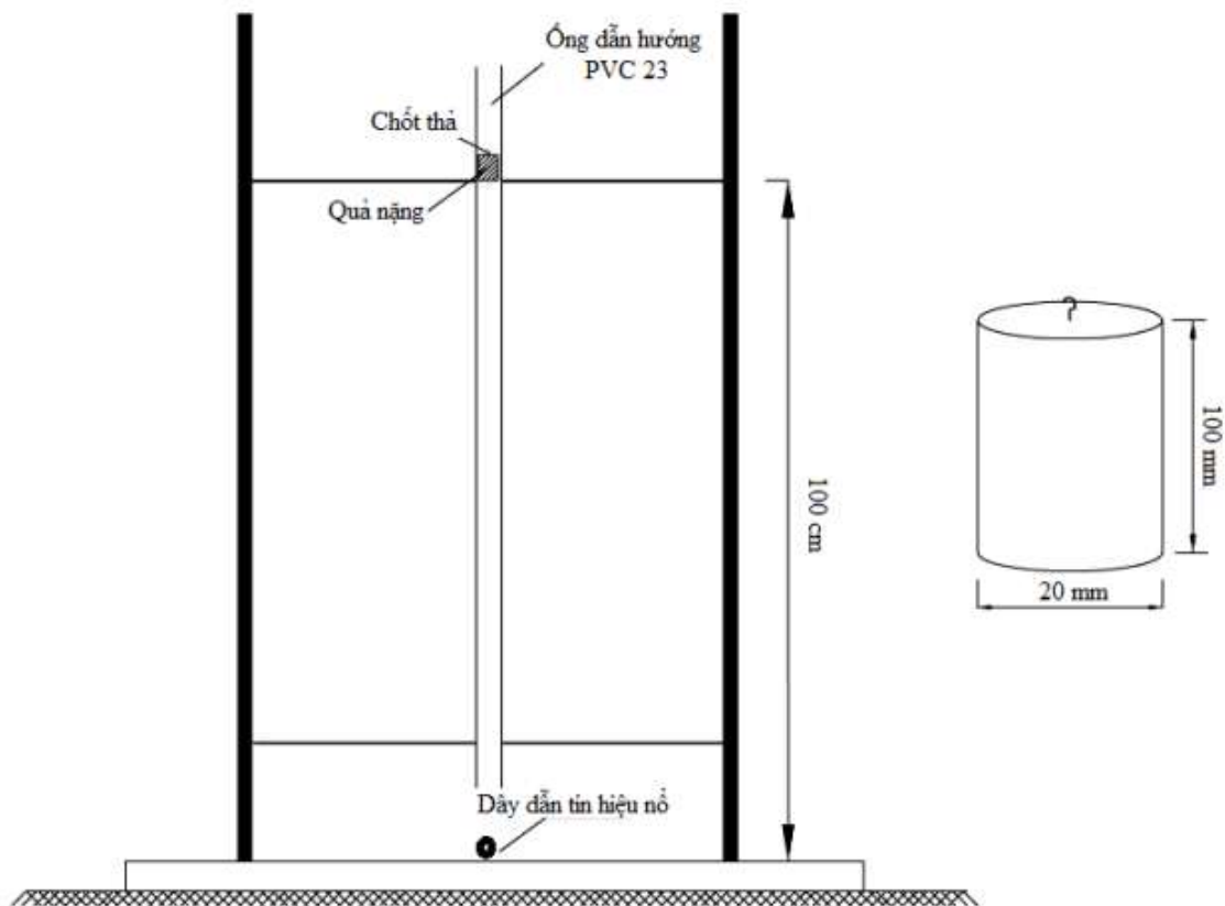
Hình 3a: Thử nghiệm độ nhảy và đập của dây dẫn tín hiệu nổ
