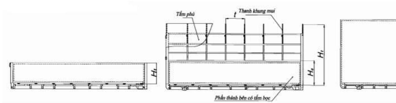
Thùng hở không mui phủ
