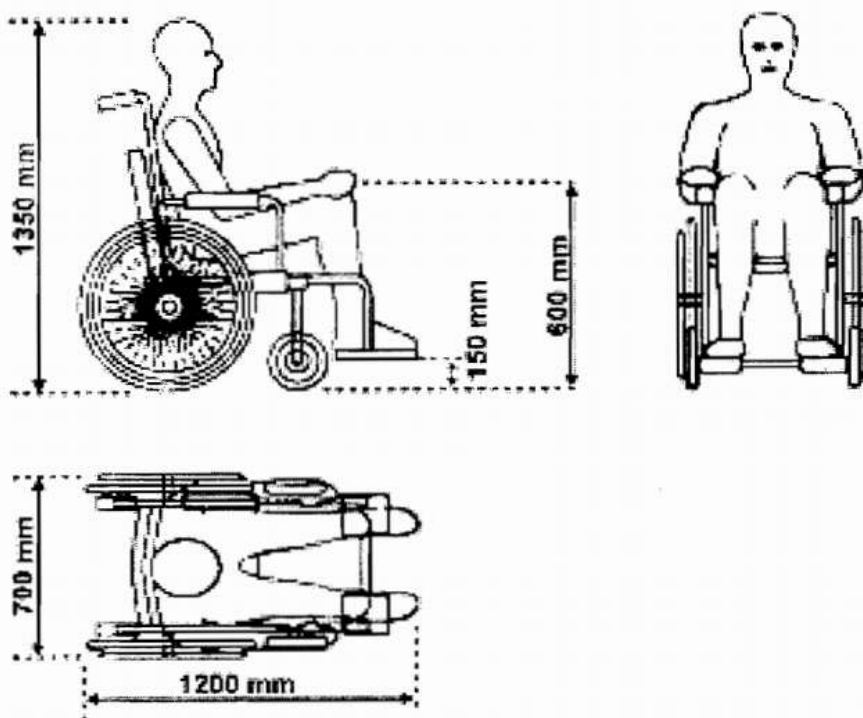
Hình 1. Xe lăn chuẩn
