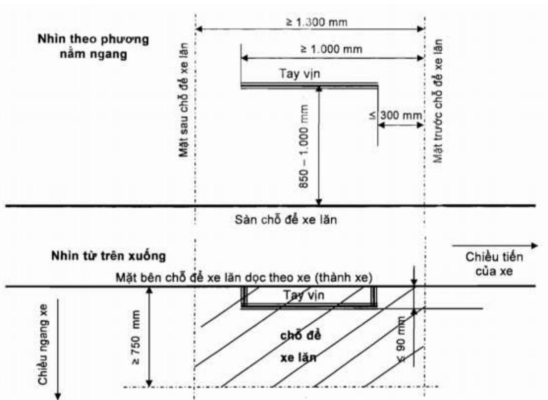
Hình 3. Bố trí tay vịn
