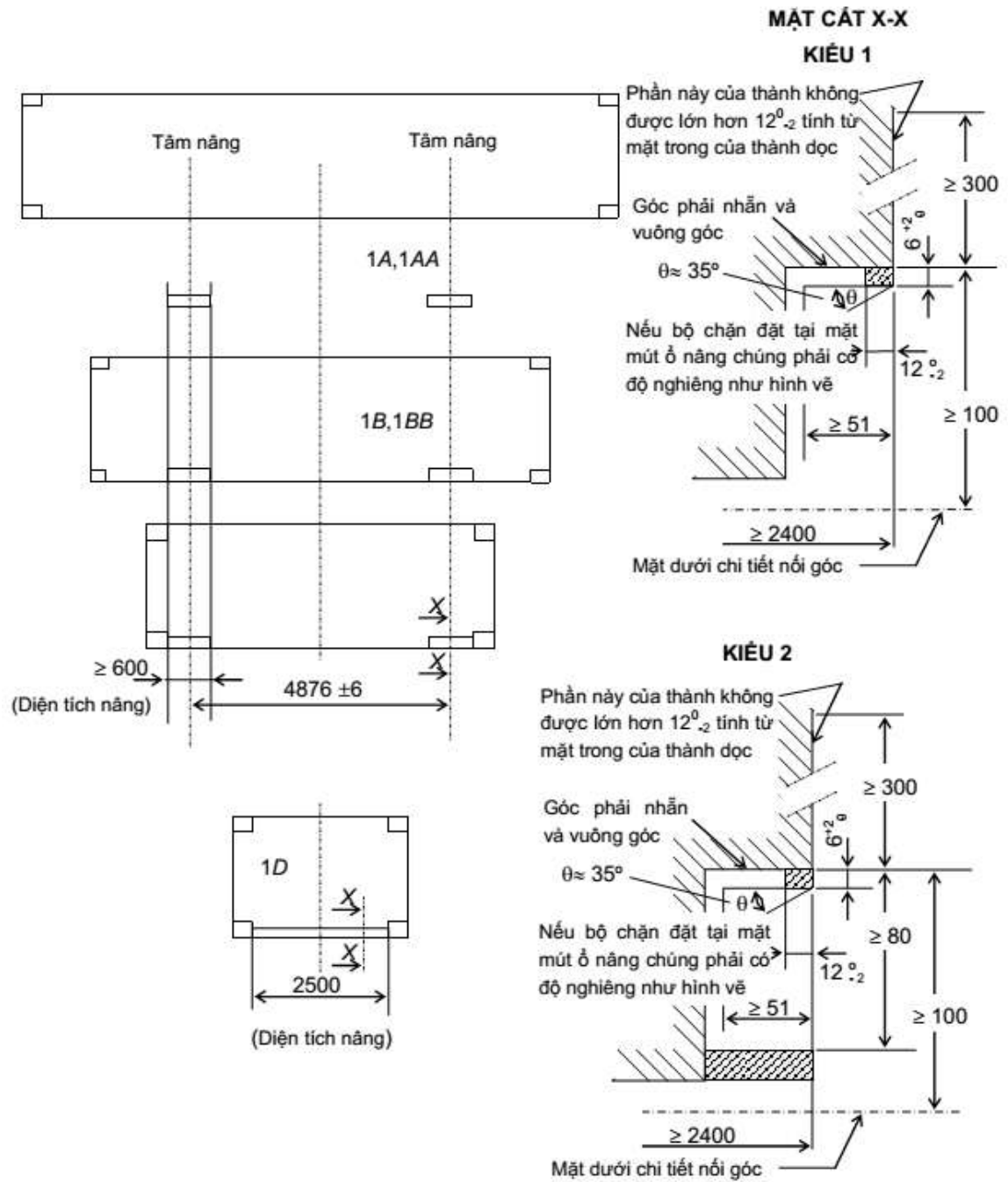
Hình 7. Vùng kẹp chạc nâng
