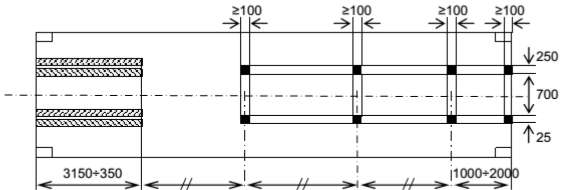
CÔNG-TE-NƠ 1A, 1AA VÀ 1AAA HOẶC 1AX CÓ RÃNH CỎ NGỔNG
