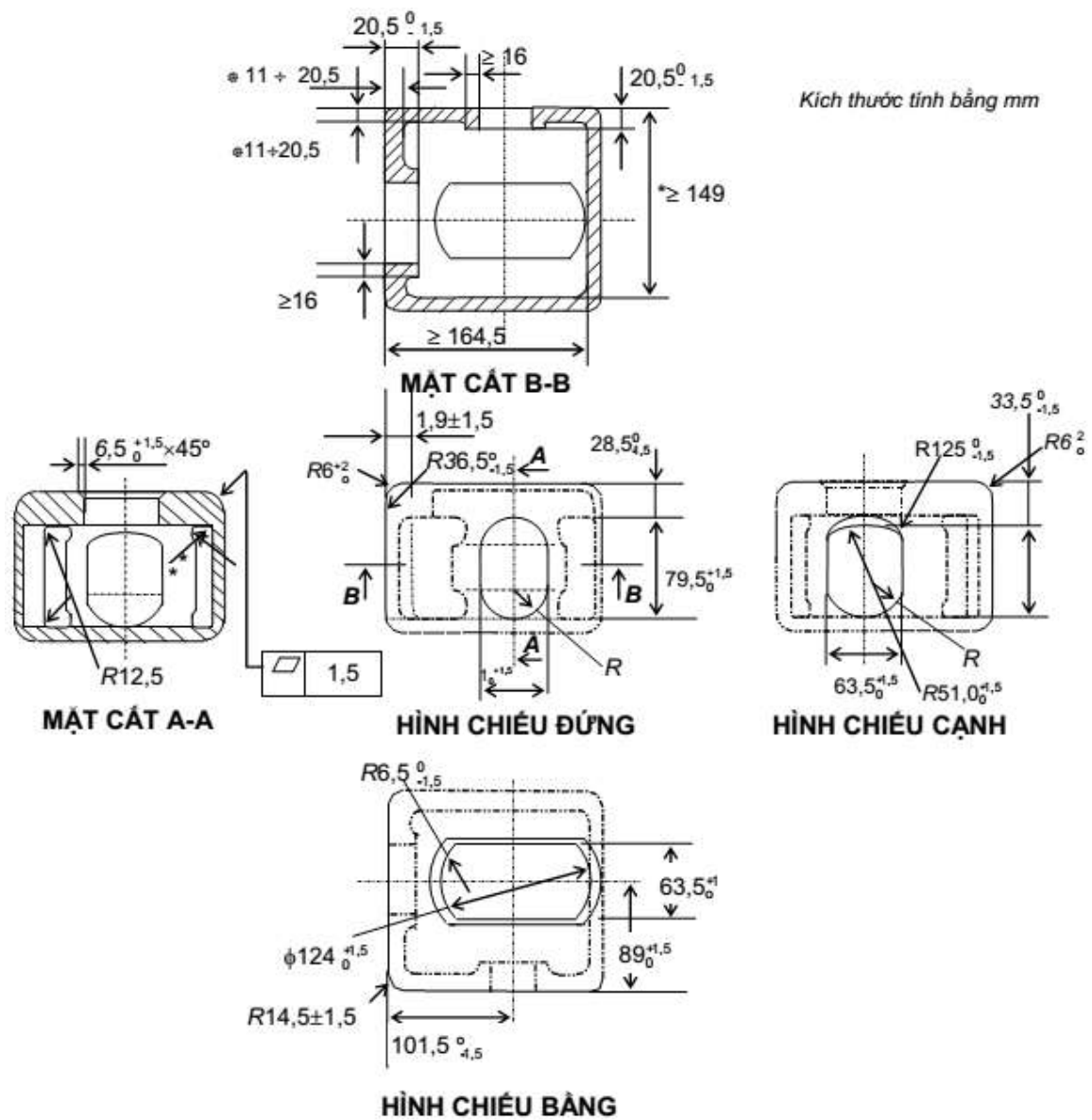
Hình 2. Chi tiết nối góc phía trên
