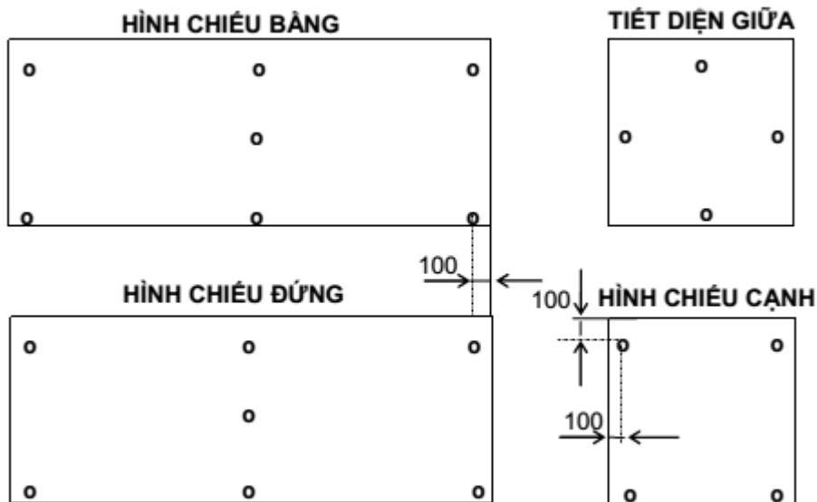
Hình 13. Điểm đo nhiệt độ không khí (bên trong và bên ngoài)
