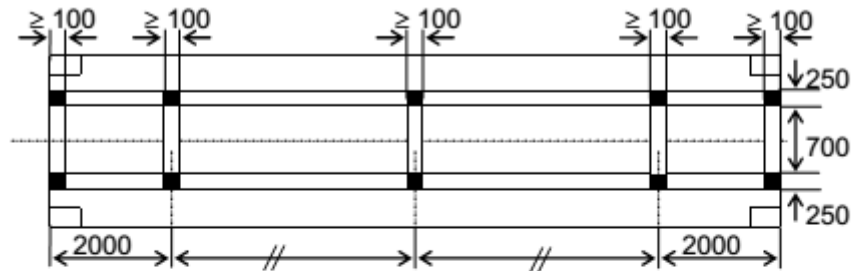
CÔNG-TE-NƠ 1A, 1AA HOẶC 1AX KHÔNG CÓ RÃNH CỎ NGỔNG
