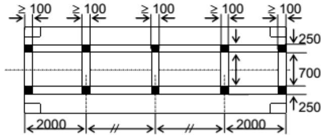
CÔNG-TE-NƠ 1B VÀ 1BB
