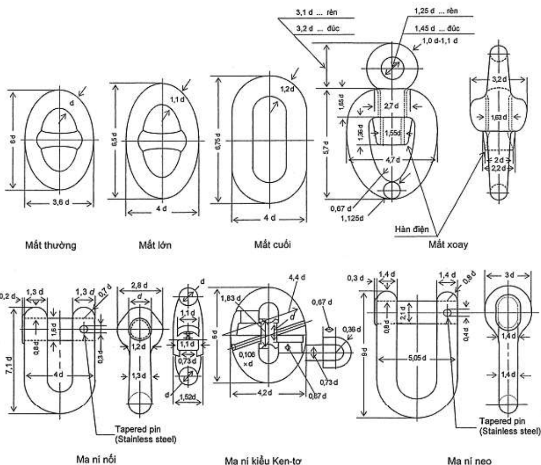
(2) Xích có ngang và ma ní
