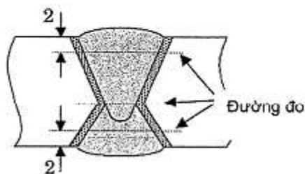
Hình 6/4.5 Thử độ cứng (đơn vị tính: mm)
