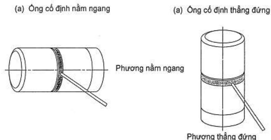
Hình 6/5.2 Tư thế hàn ống
