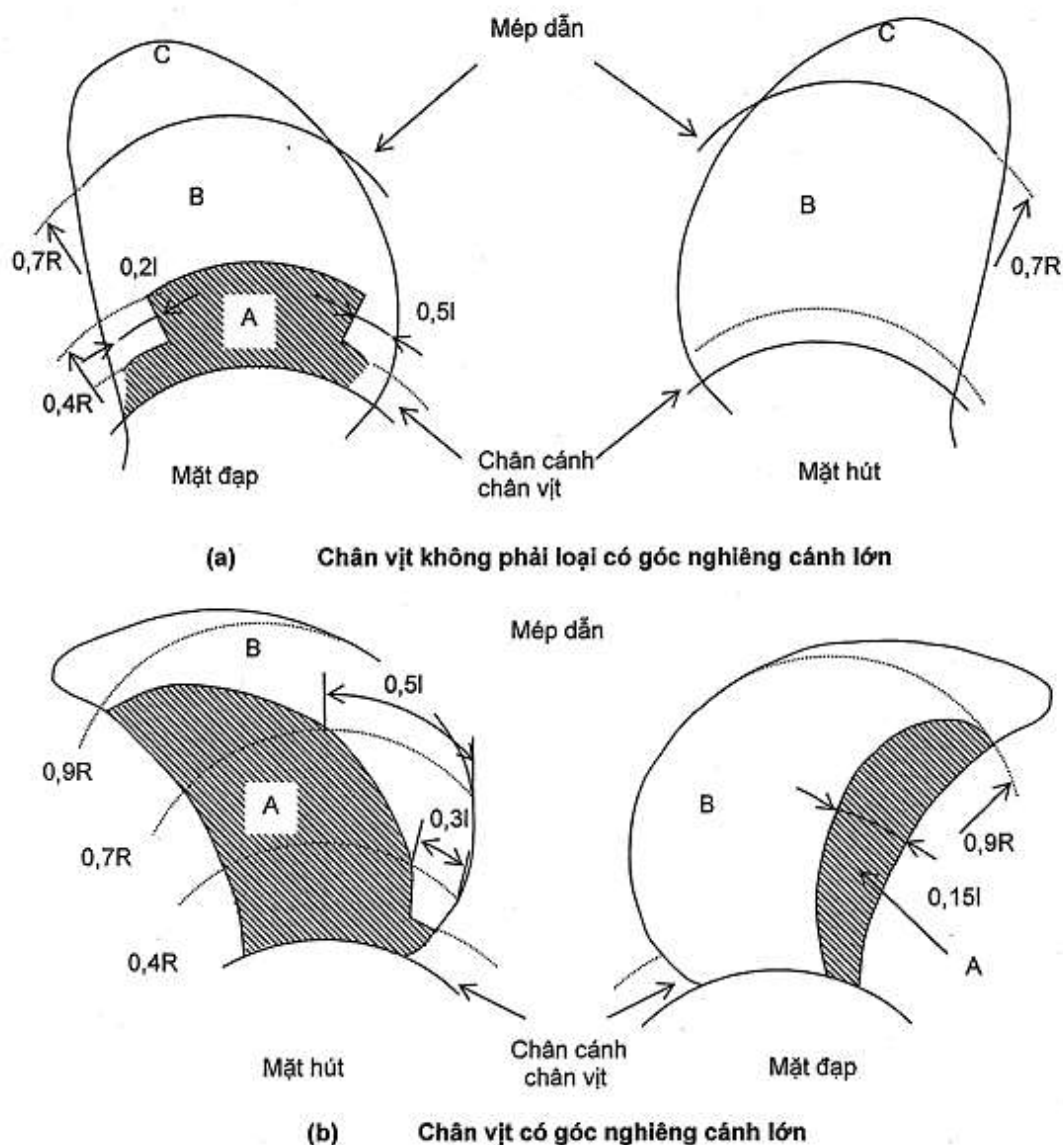
Hình 7A/7.1 Vùng quy định kiểm tra không phá hủy của đông đúc chân vịt
