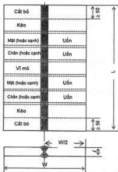
(F) Vật thử dùng cho hợp kim vật thử thử chất lượng quy trình hàn nhôm
