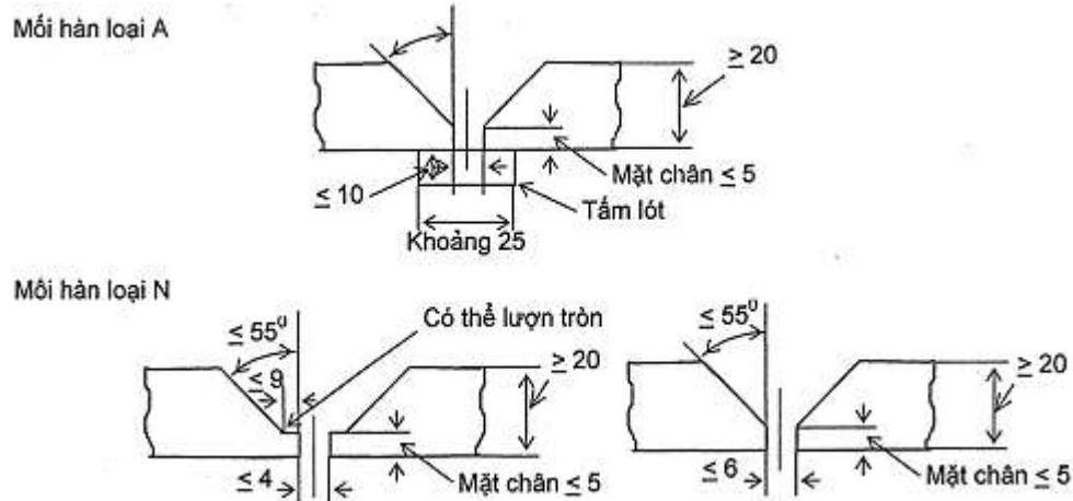
Hình 6/5.5 Kích thước và dạng của vật thử cho vật liệu tấm của thợ Bạc 3
