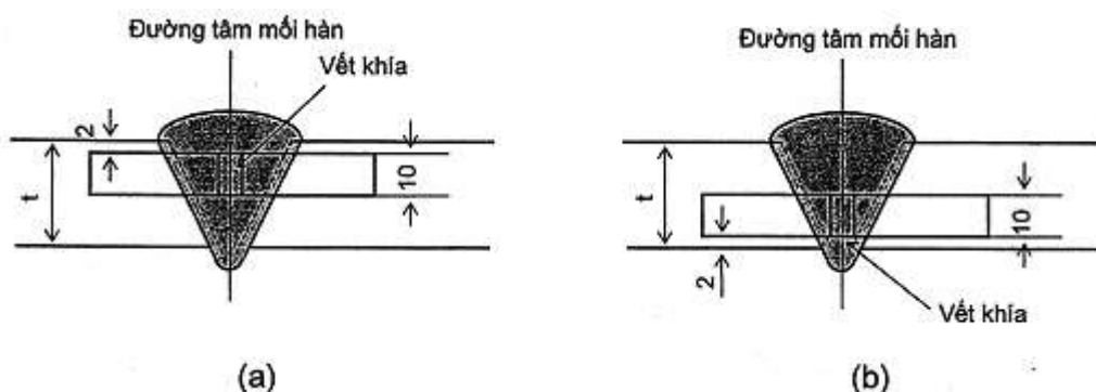
Hình 6/6.15 Vị trí mẫu thử độ dai va đập mối hàn giáp mép được hàn bằng kỹ thuật hàn nhiều lớp và một lớp
