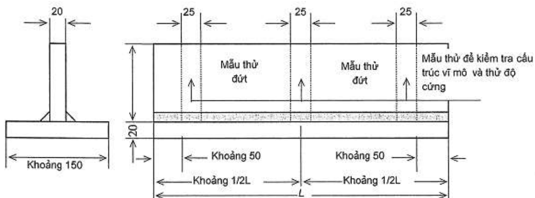
Hình 6/6.2 Vật thử mối hàn giáp mép (đơn vị: mm)
