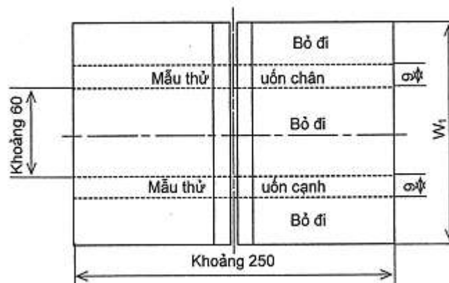
Hình 6/5.4 Kích thước và dạng của vật thử cho vật liệu tấm của Bạc 2
