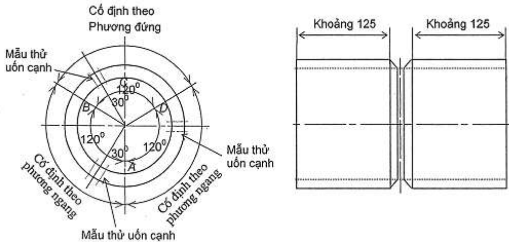
Hình 6/5.7 Kích thước và dạng của vật thử hình ống của thợ Bạc 2
