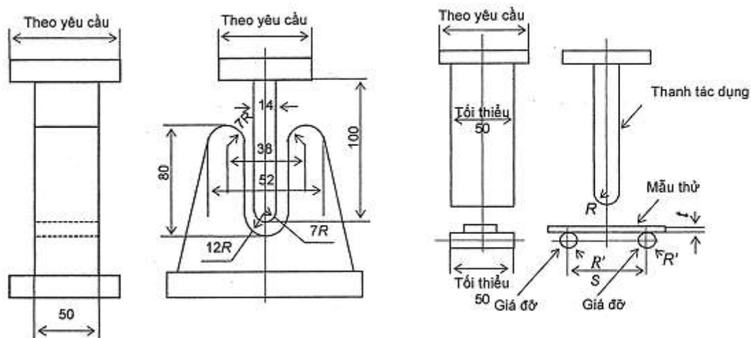
Hình 6/3.2 Đồ gá để thử uốn có rãnh dẫn hướng
