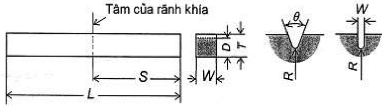
Hình 7A/2.1 Mẫu thử độ dai va đập
