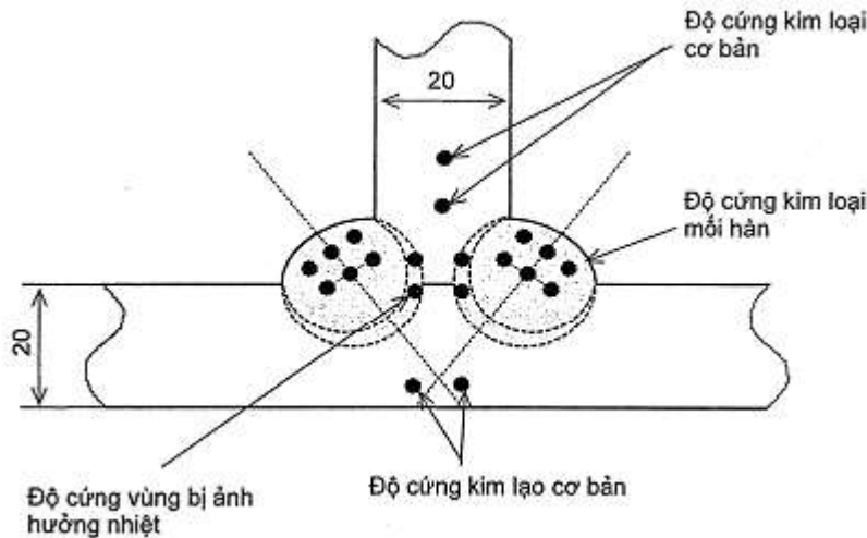
Hình 6/6.5 Thử độ cứng (đơn vị: mm)
