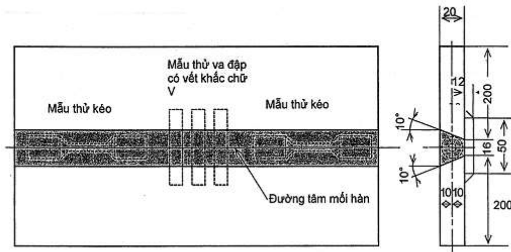
Hình 6/6.7 Vật thử kim loại đắp với kỹ thuật hàn nhiều lớp (đơn vị: mm)
