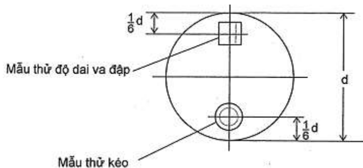
Hình 7A/3.2 Chọn mẫu thử
