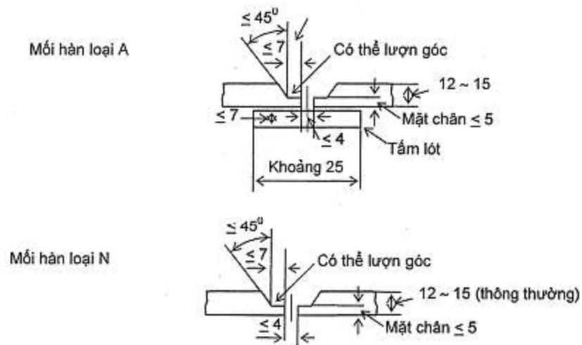
Hình 6/5.7 Kích thước và dạng của vật thử hình ống của thợ Bạc 2
