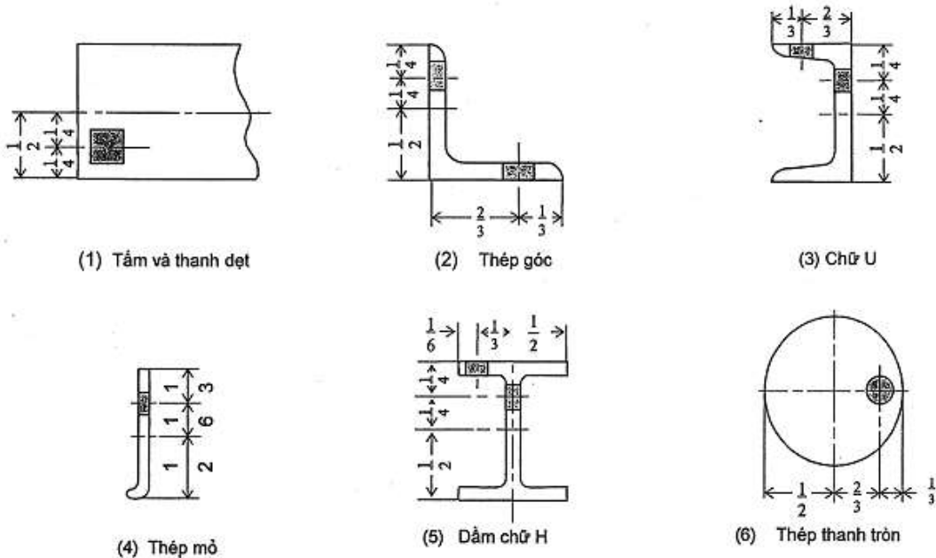
Hình 7A/3.1 Chọn vật mẫu
