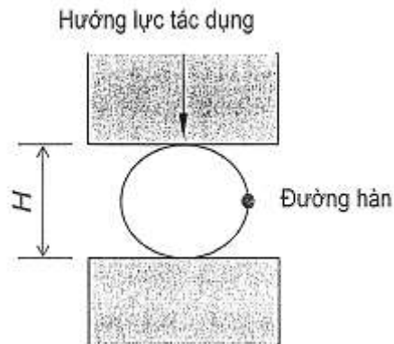
Hình 7A/4.1 Thử làm bẹp
