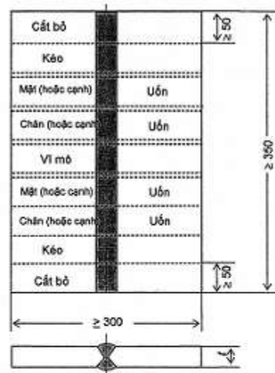
(E) Vật thử dùng cho thép tấm không gỉ
