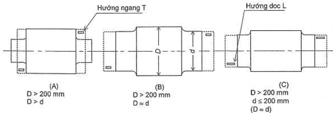
Hình 7A/6.4 Chọn mẫu thử đối với bánh răng có đường kính lớn hơn 200 mm
