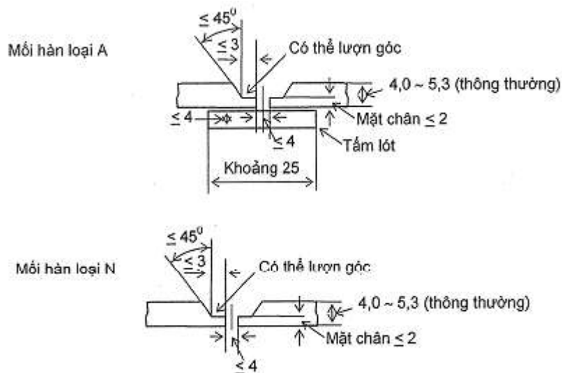
Hình 6/5.6 Kích thước và dạng của vật thử hình ống của thợ Bạc 1
