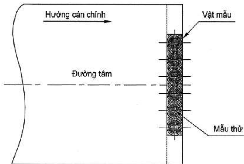
Hình 7A/3.4 Chọn vật mẫu thử
