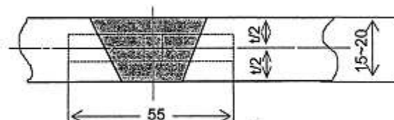
Hình 6/6.4 Vị trí của mẫu thử va đập
