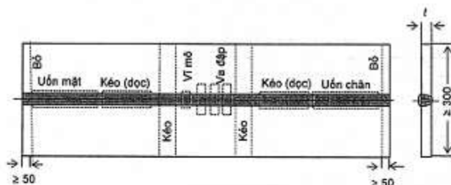
(D) Vật thử dùng cho vật liệu L9N53 hoặc L9N60
