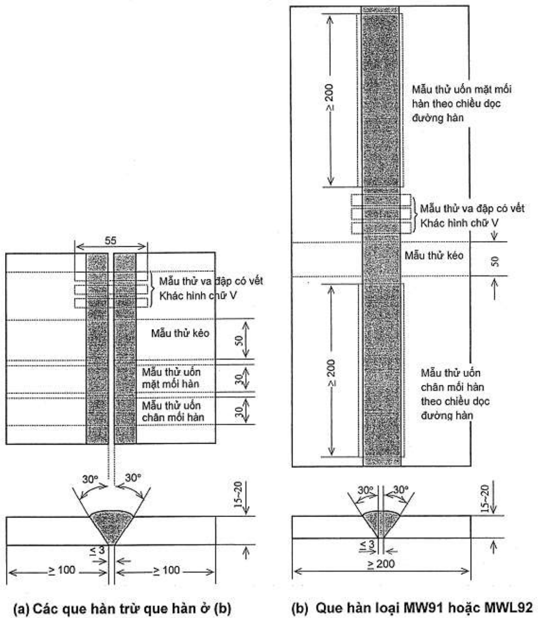
Hình 6/6.2 Vật thử mối hàn giáp mép (đơn vị: mm)
