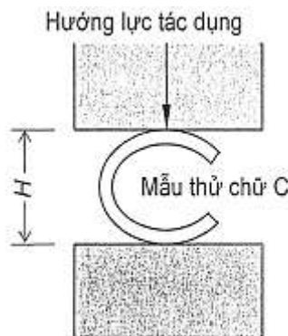
Hình 7A/4.2 Thử làm bẹp cho mẫu thử chữ C
