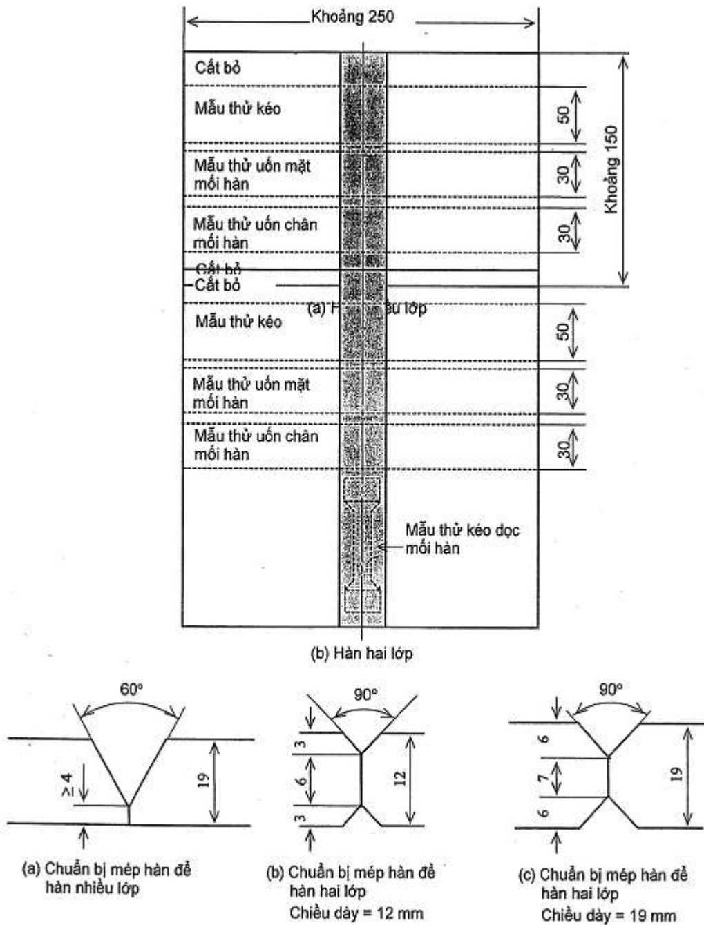
Hình 6/6.18 Vật thử mối hàn giáp mép đối với hàn hồ quang dưới thuốc (đơn vị: mm)
