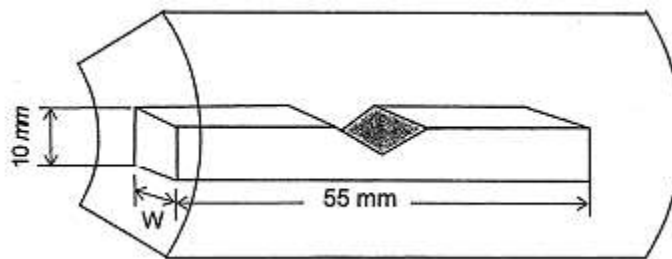
Hình 7A/4.3 Vị trí chọn mẫu thử độ dai và đập cắt từ ống liền hoặc ở những chỗ không thuộc đường hàn từ ống làm bằng phương pháp hàn điện trở
