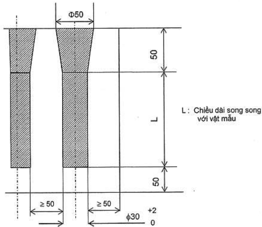
Hình 7A/5.1 Mẫu thử (Đơn vị: mm)
