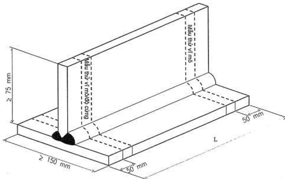
Hình 6/4.8 Vật thử cho mối hàn chữ T ngấu toàn bộ
