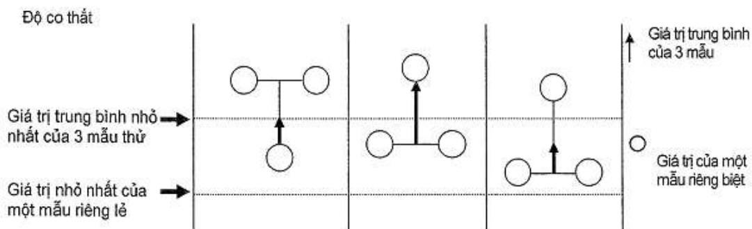
Hình 7A/3.5 Kết quả thử lại cho phép
