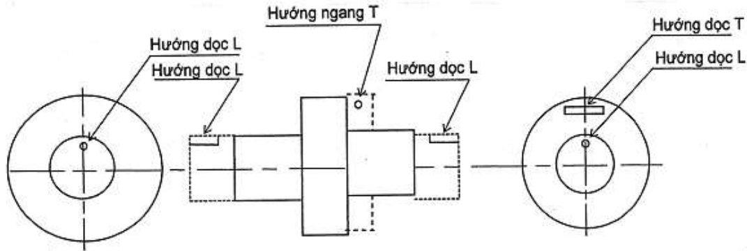
Hình 7A/6.1 Chọn mẫu thử đối với rôto tua bin
