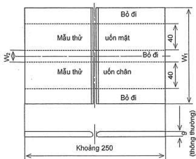
Hình 6/5.3 Kích thước và dạng của vật thử cho vật liệu tấm của Bạc 1
