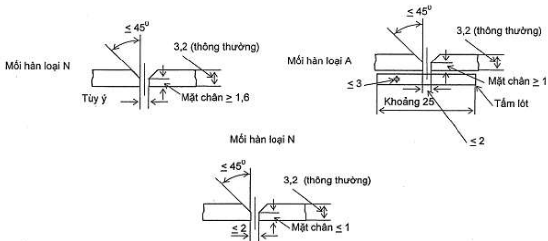
Hình 6/5.3 Kích thước và dạng của vật thử cho vật liệu tấm của Bạc 1
