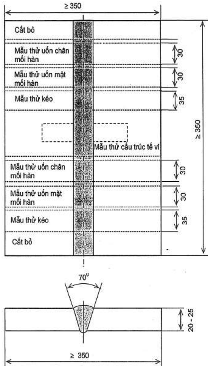
Hình 6/6.20 Vật thử mối hàn giáp mép có chiều dày từ 10-12 (đơn vị: mm)
