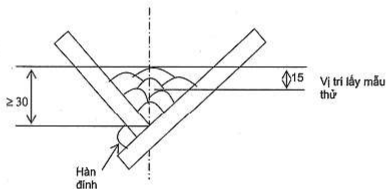
Hình 6/6.19 Vật thử kim loại đắp (đơn vị: mm)
