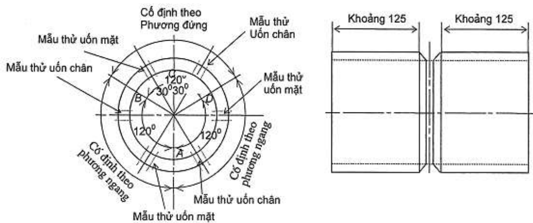
Hình 6/5.6 Kích thước và dạng của vật thử hình ống của thợ Bạc 1
