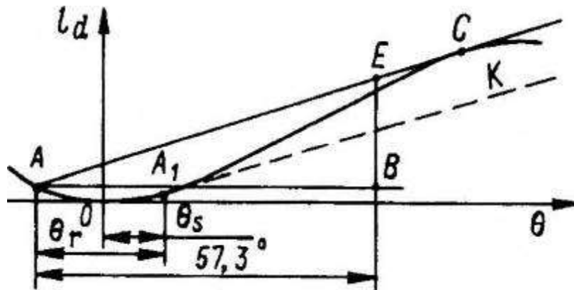
Hình 10/Phụ lục 1/1.2.1 Xác định mô men lật của cần cầu nổi ở trạng thái chòng chành khi đi biển theo đường cong ổn định động.
