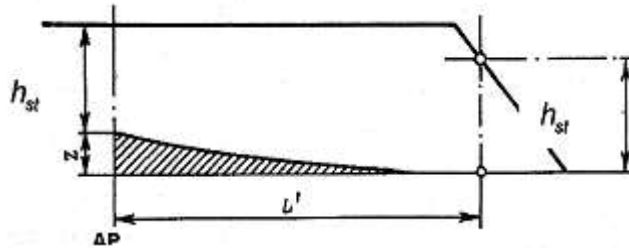
Hình 11/4.3.4-3 Thượng tầng có vách nghiêng
