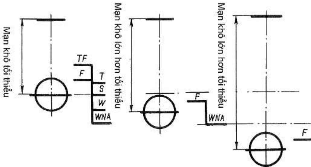
Hình 11/2.2.5 Dấu chở hàng của tàu có mạn khô lớn hơn mạn khô tối thiểu
