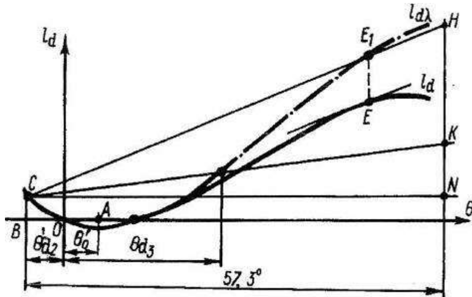
Hình 10/Phụ lục 1/1.1 Xác định mô men lật và góc nghiêng động khi hàng bị rơi
