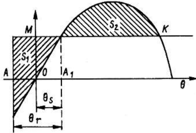
Hình 10/Phụ lục 1/1.2.2 Xác định mô men lật của cần cẩu nổi ở trạng thái chẳng giữ khi đi biển theo đường cong ổn định tĩnh
