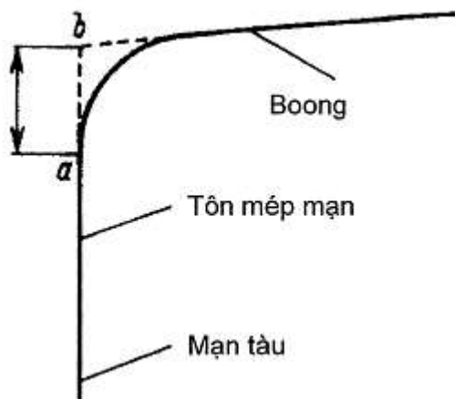
Hình 11/2.1.1-2 Vị trí đường boong của boong lượn tròn
