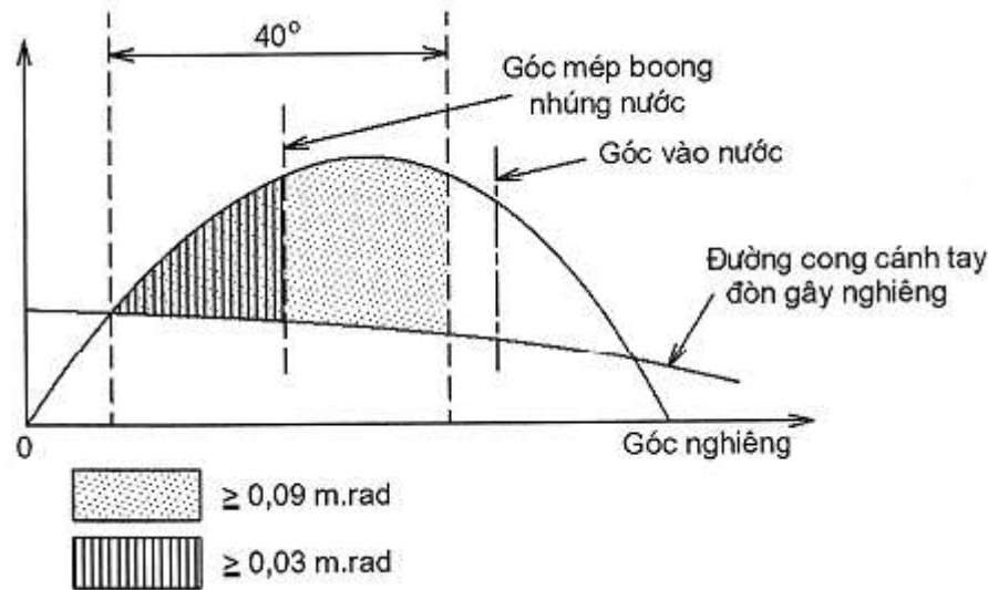
Hình 10/3.11 Diện tích giữa cánh tay đòn hồi phục và cánh tay đòn gây nghiêng CHƯƠNG 4 YÊU CẦU ỔN ĐỊNH CỦA CẦN CẦU NỔI, TÀU CẦU, PHAO CHUYỂN TẢI, Ụ NỔI VÀ BẾN NỔI
