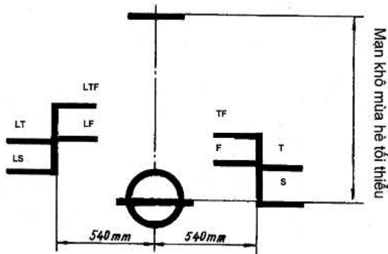
Hình 11/6.2.3-2 Đường nước chở hàng tàu hoạt động ở vùng hạn chế
