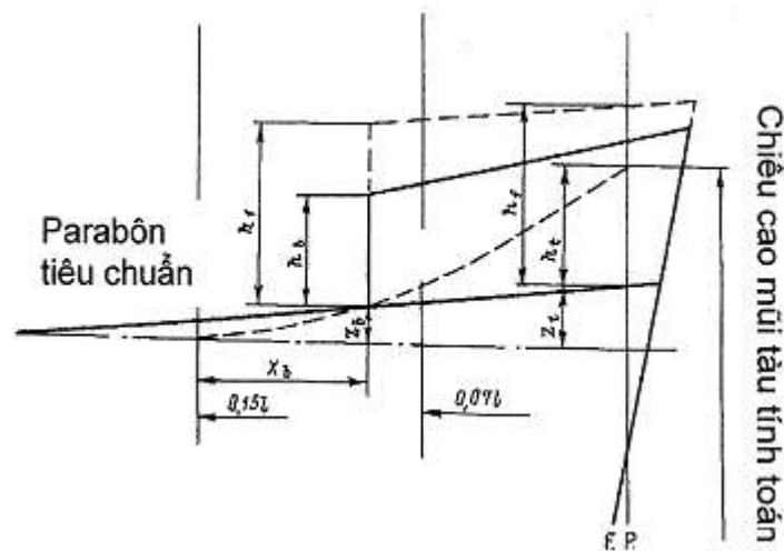
Hình 11/4.4.8-4(1) Độ cong dọc kéo dài ngoài phạm vi 0,15L
