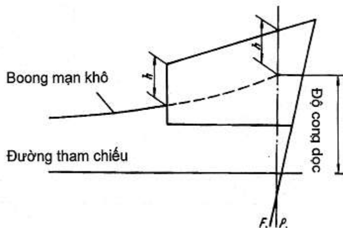
Hình 11/4.3.1-6 Độ cong dọc khi có thượng tầng mũi
