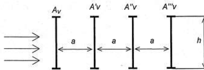
Hình 4.1.5-1 (3) Diện tích của các thanh che nhau
