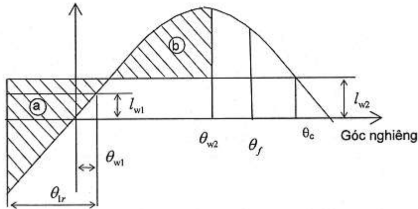
Hình 2.1.2-1 Ổn định thời tiết
