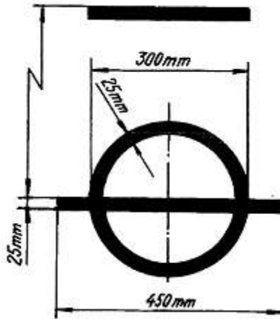
Hình 11/2.1.2 Dấu mạn khô
