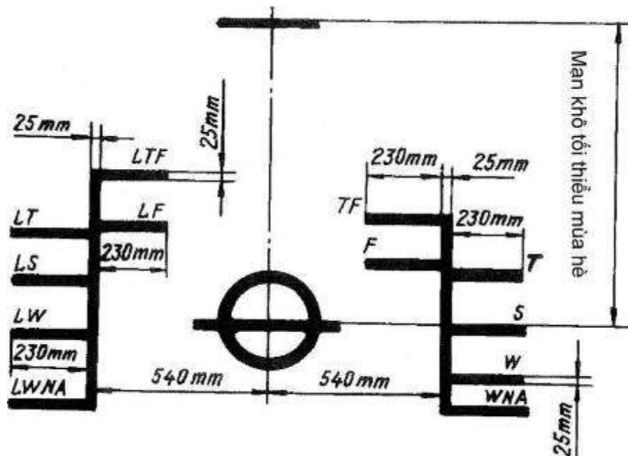
Hình 11/2.2.1 Dấu đường nước chở hàng
