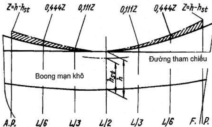
Hình 11/4.3.1.1-5 Thượng tầng kéo dài suốt chiều dài tàu
