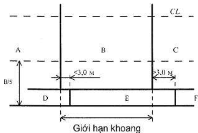
Hình 9/4.3.5-1 Giả định ngập
