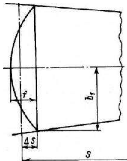
Hình 11/4.2.2-2 Vách mút thượng tầng nhô ra
