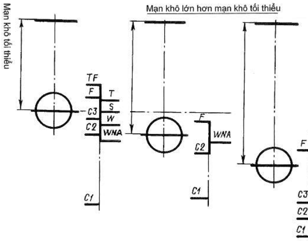
Hình 11/2.2.6-2 Dấu đường nước chờ hàng
