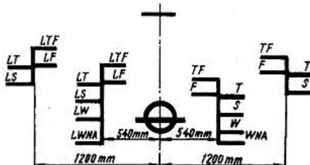
Hình 11/6.2.4-1(1) Mạn khô kép
