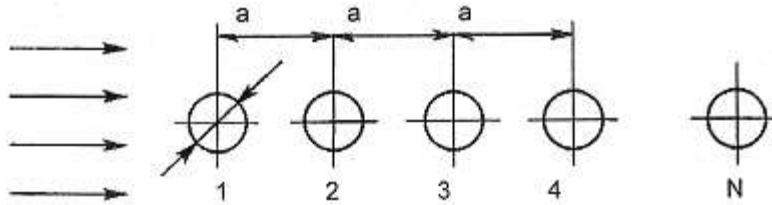
Hình 4.1.5-1(4)(a) Diện tích của các dây che nhau
