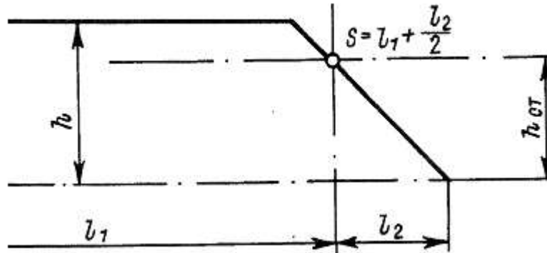
Hình 11/4.2.2-4(1) Vách mút nghiêng có chiều cao nhỏ hơn tiêu chuẩn
