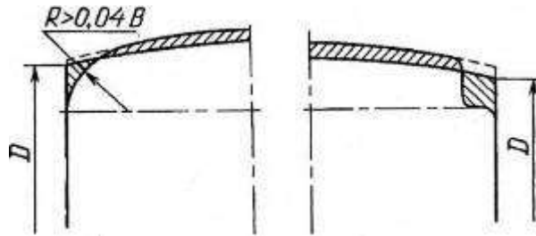
Hình 11/1.2.1 Xác định chiều cao tính mạn khô
