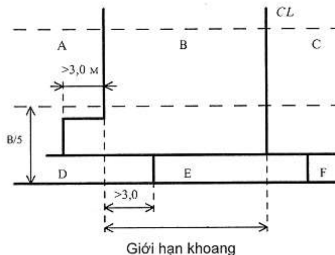
Hình 9/4.3.5-4 Giả định ngập
