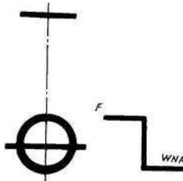
Hình 11/2.2.3 Dấu mạn khô tàu buồm
