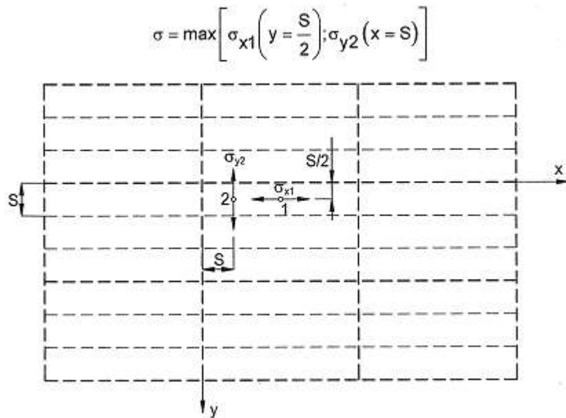
Hình 2A/18.2 Xác định ứng suất pháp trên tấm nắp miệng khoang
