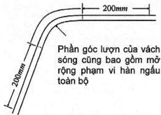
(b) Kiểu vách sóng uốn
