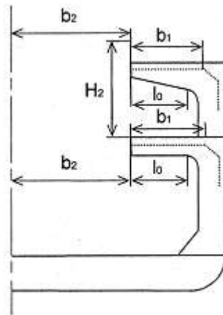
Hình 2A/5.3 Đo l_0 , b_1 , b_2 và H_2
