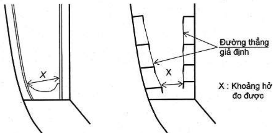
Hình 2A/29.13 Khoảng cách trong lòng giữa các kết cấu trong mạn kép
