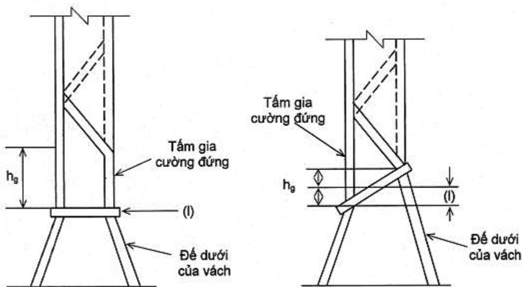
Hình 2A/29.8b Tấm gia cường đứng
