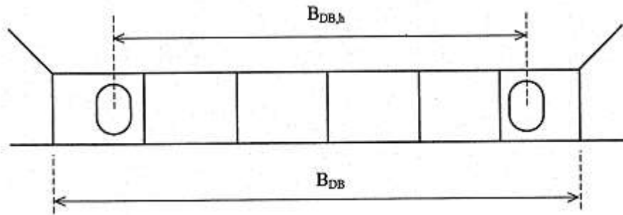
Hình 2A/29.12 Xác định B_{DB} và B_{DB,h}
