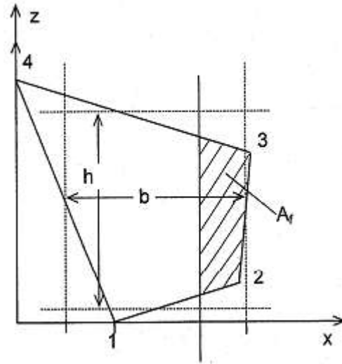
Hình 2B/21.1.2 Hệ thống tọa độ của bánh lái
