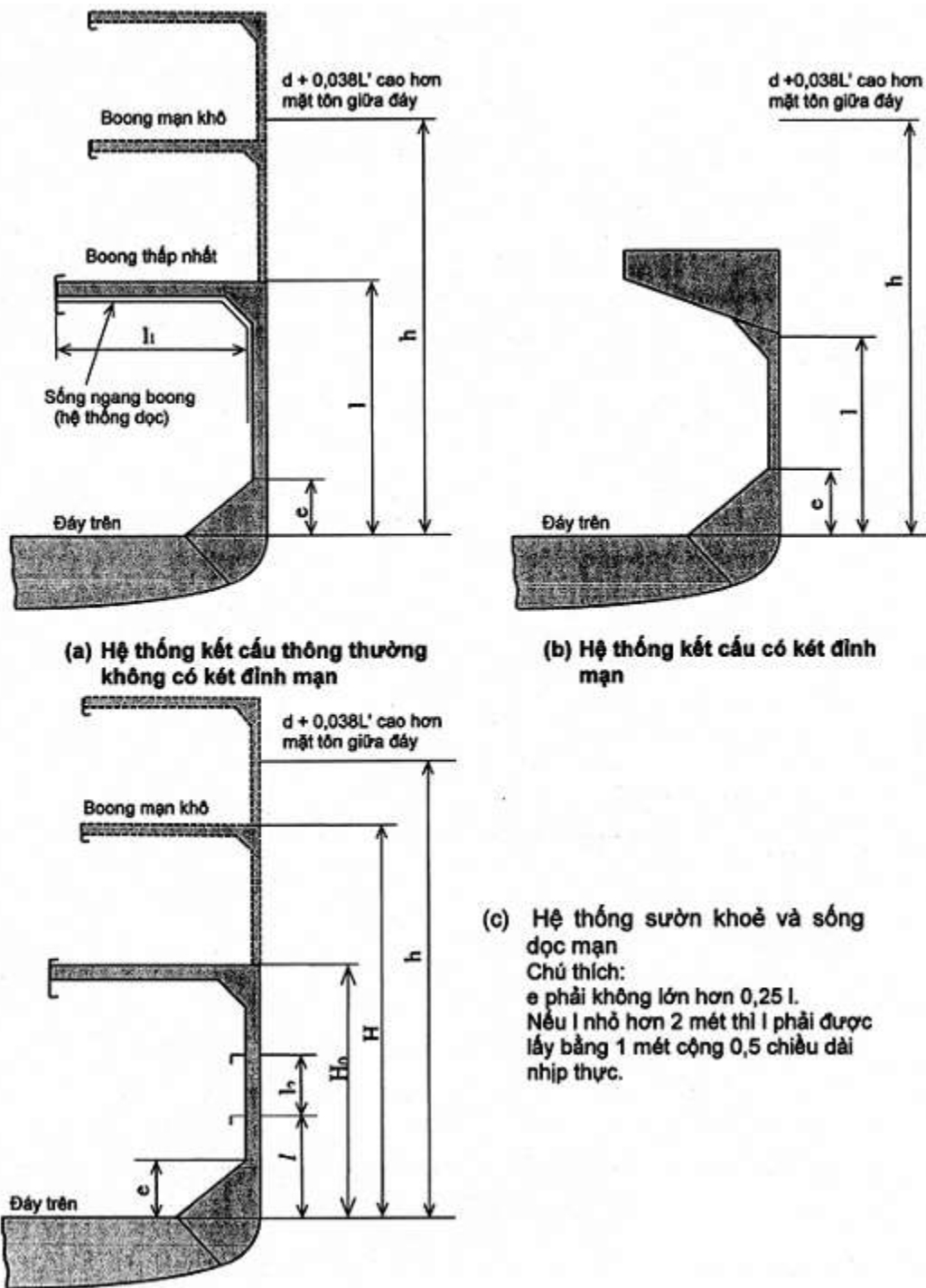
Hình 2A/5.2 l , h , H v.v... dùng cho sườn khoang
