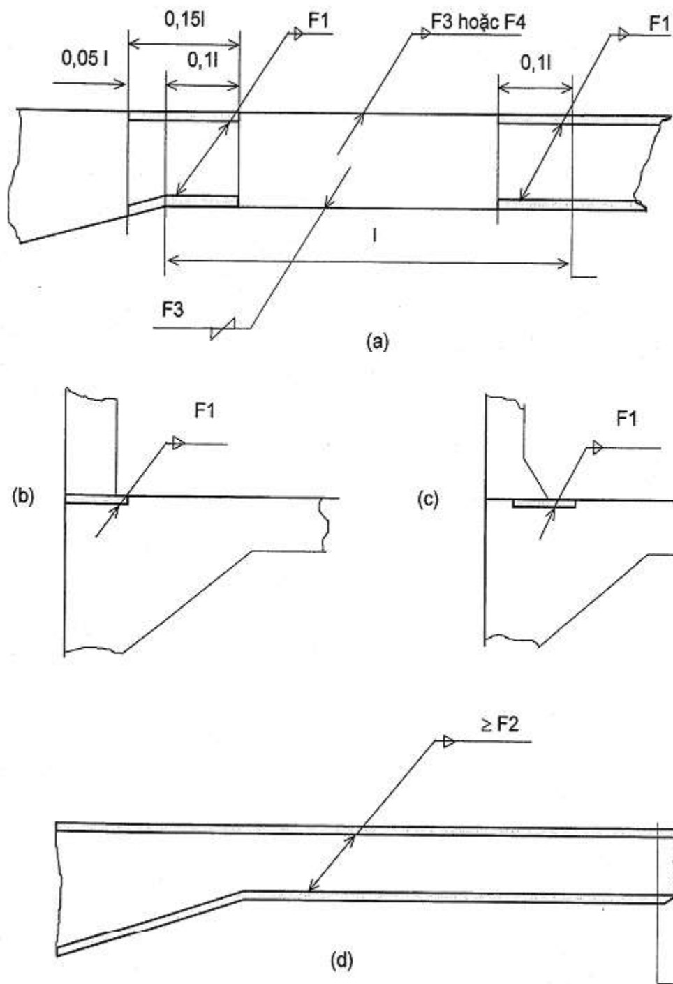
Hình 2A/1.3 Phần liên tục của đường hàn CHƯƠNG 2 SÓNG MŨI VÀ SÓNG ĐUÔI
