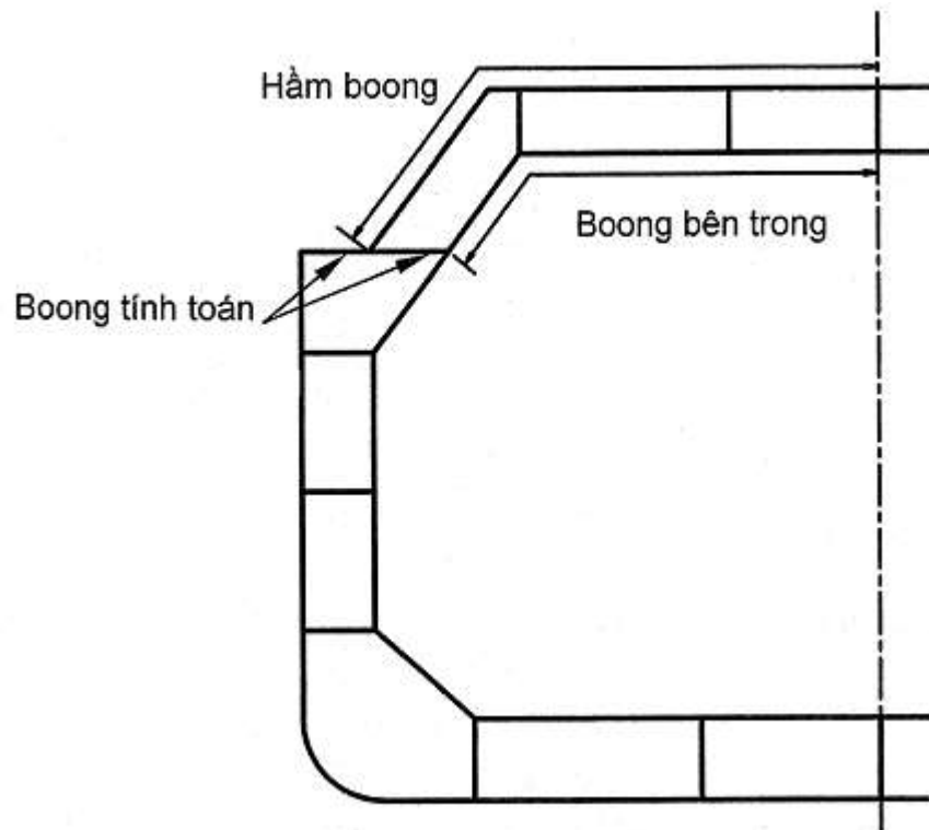
Hình 2A/1.2 Đặc trưng kết cấu boong của tàu chở xô khí hóa lỏng
