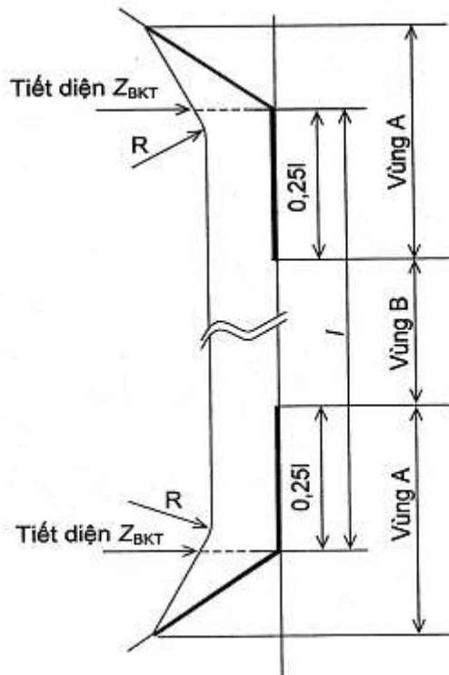
Hình 2A/29.3 Sườn khoang và các mã nút
