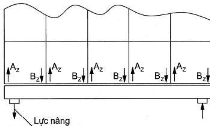
Hình 2A/18.9 Lực nâng trên nắp khoang hàng
