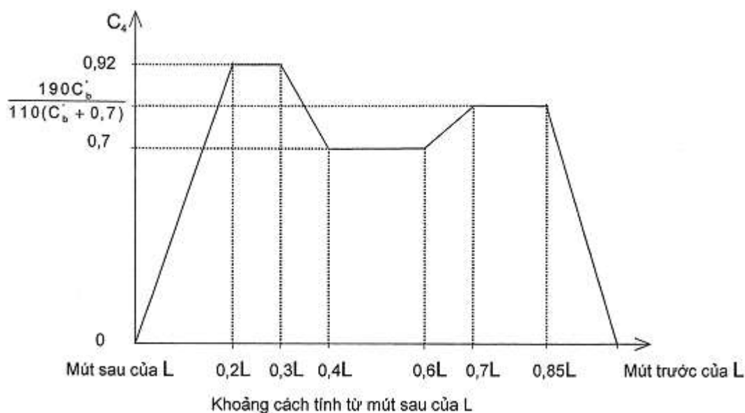
Hình 2A/13.5 Trị số của hệ số C_4
