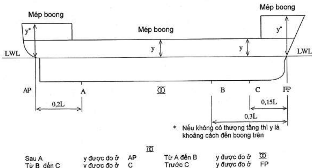
Hình 2B/15.1 Vị trí đo y
