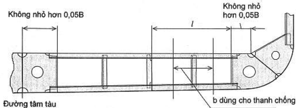
Hình 2A/4.1 Dàn ngang hồ
