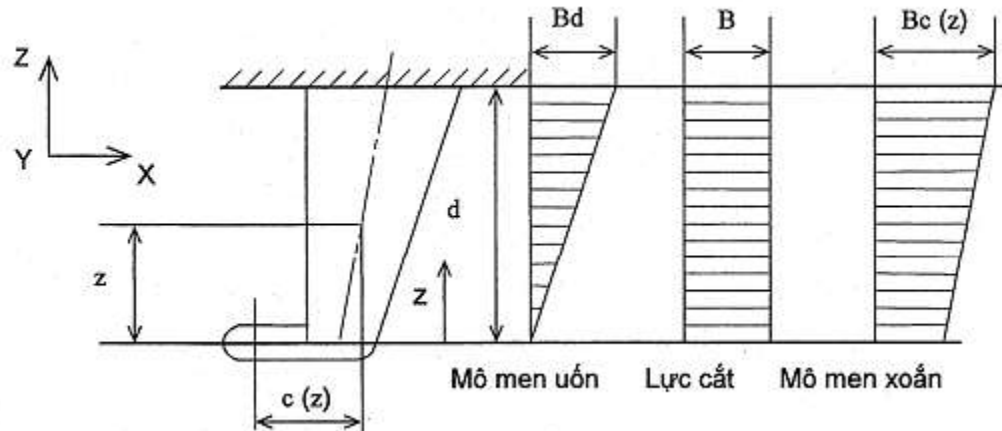
Hình 2A/2.3 Giá bánh lái
