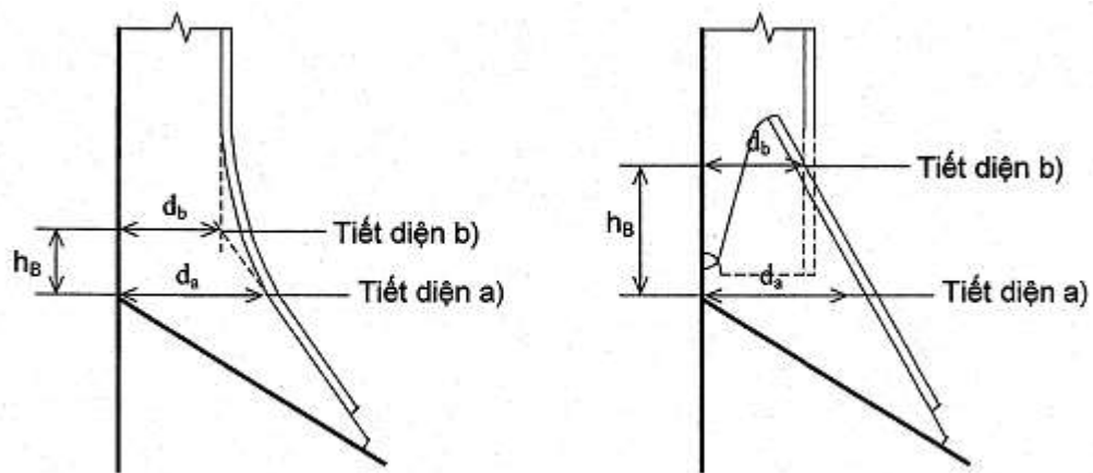
Hình 2A/29.14 Phần dưới và các vùng của sườn
