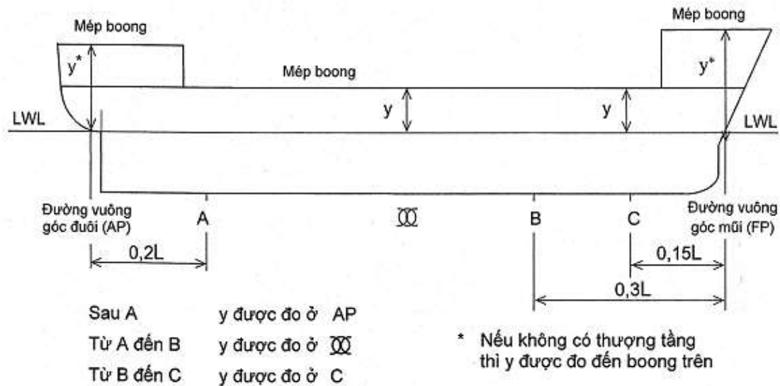
Hình 2A/8.2 Vị trí đo y
