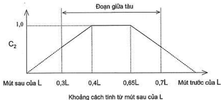
Hình 2A/13.2 Trị số của hệ số C 2
