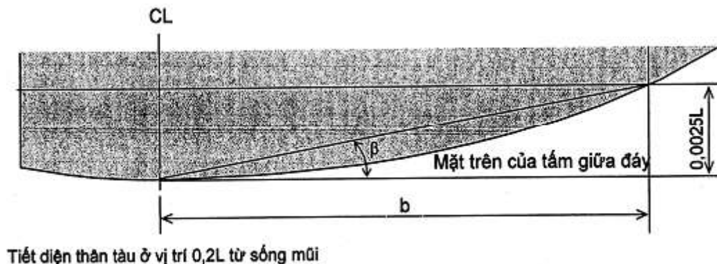
Hình 2B/4.2 Cách đo b
