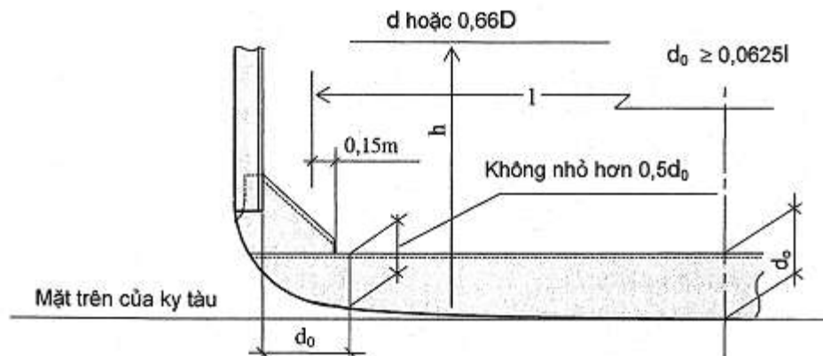
Hình 2B/3.1 Hình dạng của đà ngang đáy
