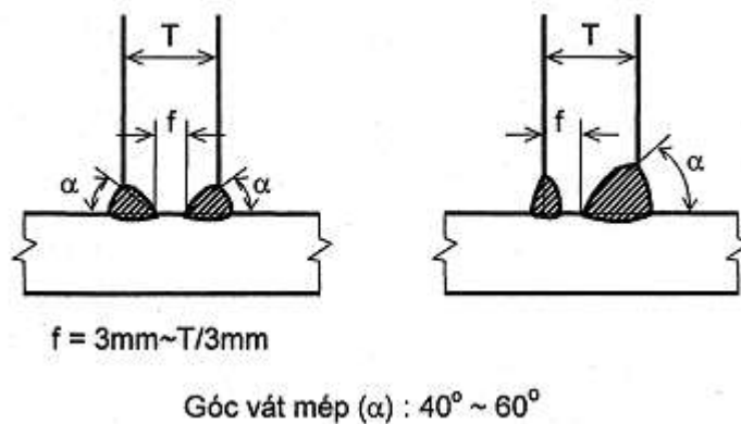
Hình 2A/29.10 Yêu cầu đối với mối hàn
