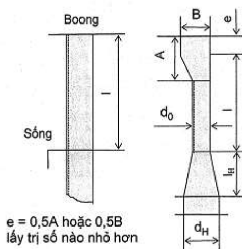
Hình 2A/11.3 Đo l
