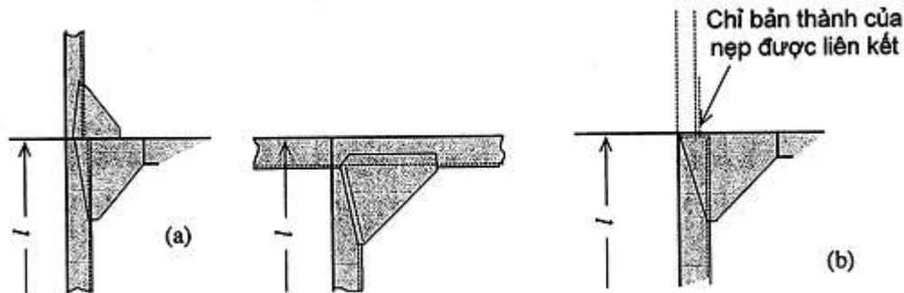
Hình 2B/11.1 Các kiểu liên kết nút
