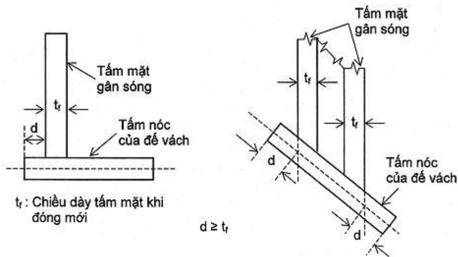
Hình 2A/29.9 Khoảng cách quy định
