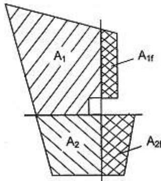
Hình 2A/25.3 Phân chia bánh lái
