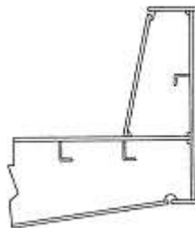
Hình 2A/18.8 Ví dụ về sự kéo dài của tấm thành miệng khoang
