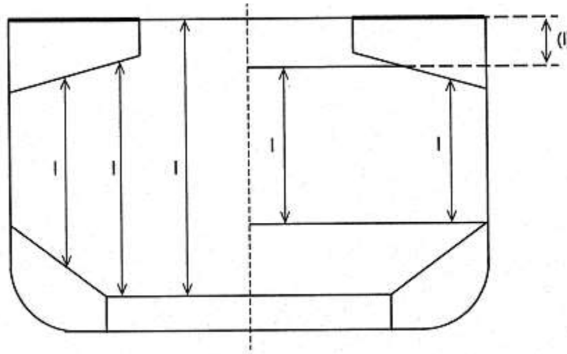
Hình 2A/29.6b Nhịp gân sóng
