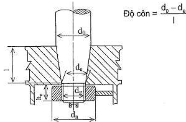
Hình 2B/21.1.4 Mối nối dạng côn
