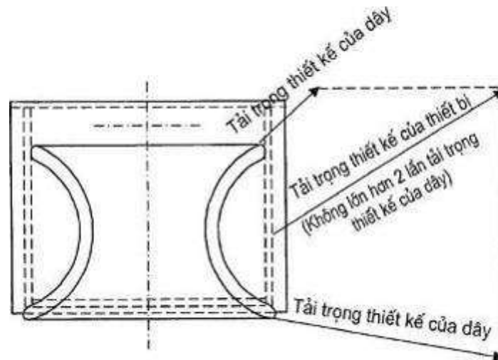
Hình 2B/21.1 Tải trọng thiết kế
