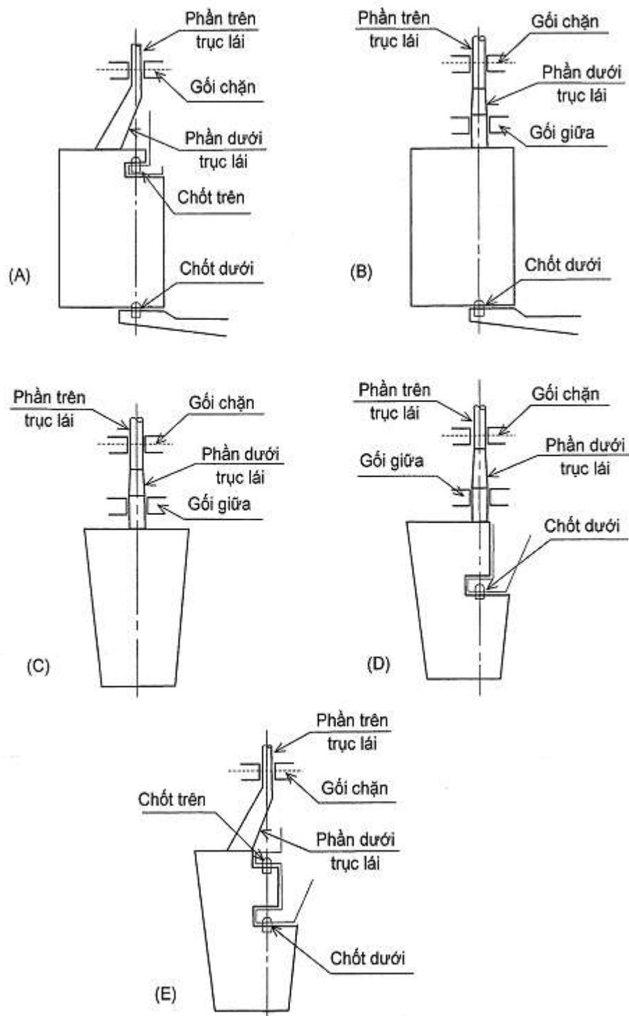
Hình 2A/25.1 Các dạng bánh lái
