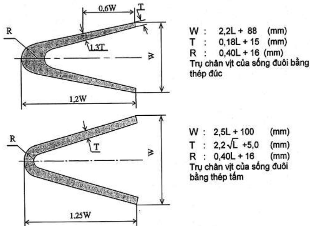
Hình 2 B/2.1 Tiêu chuẩn kích thước của trụ chân vịt
