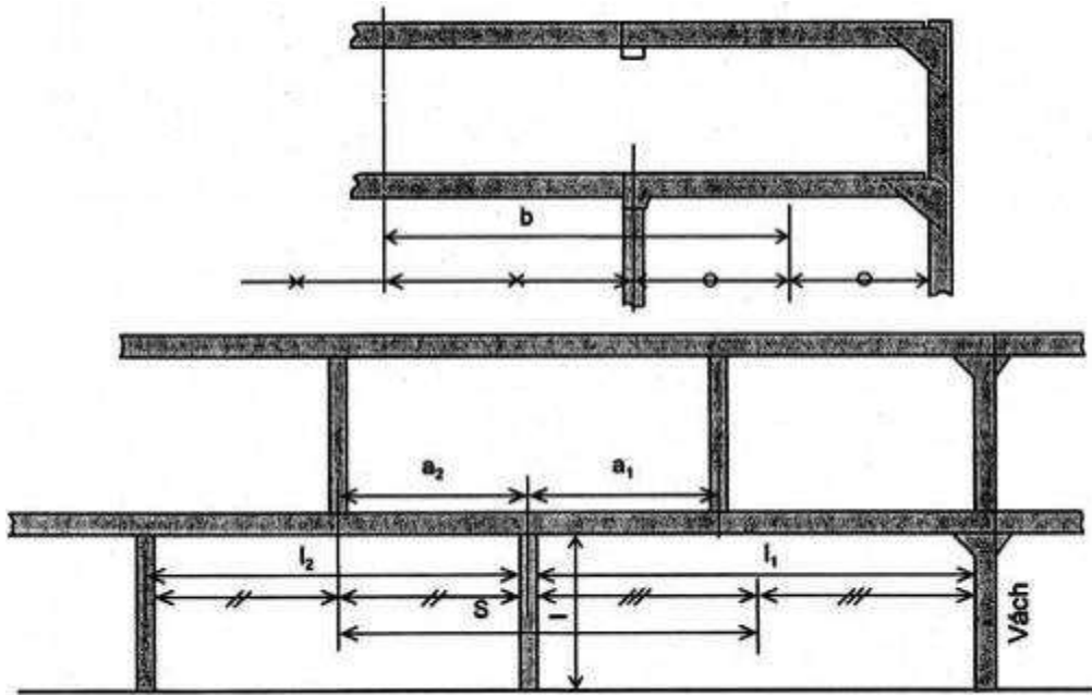
Hình 2A/9.1 Đo S, b, l,...
