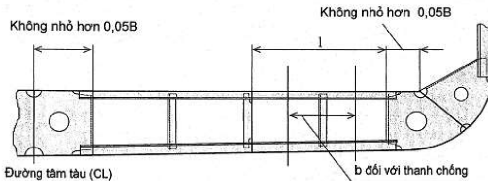
Hình 2B/4.1 Đà ngang hờ
