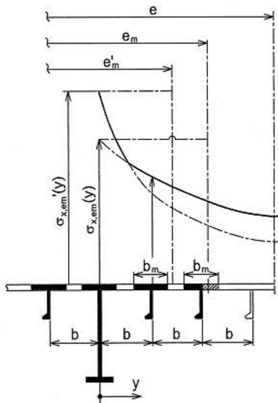
Hình 2A/18.5 Nẹp đặt song song với bản thành của cơ cấu đỡ chính
