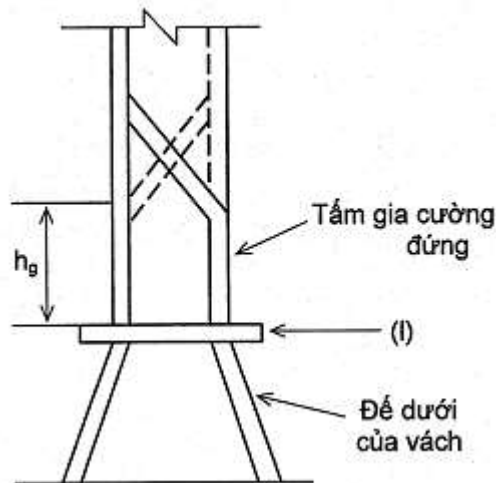
Hình 2A/29.8a Tấm gia cường đứng
