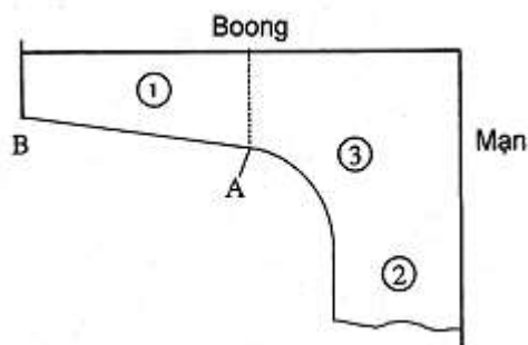
Hình 2B/6.1 Xà ngang công xon và mã đầu sườn
