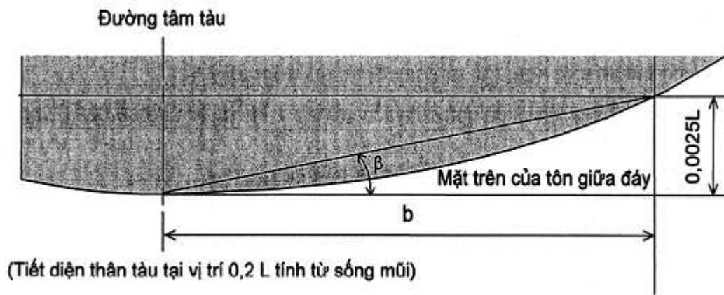
Hình 2A/4.2 Cách đo b
