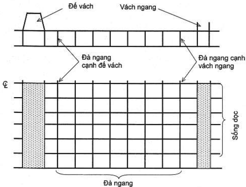
Hình 2A/29.11 Các đà ngang và sống dọc phải được tính toán
