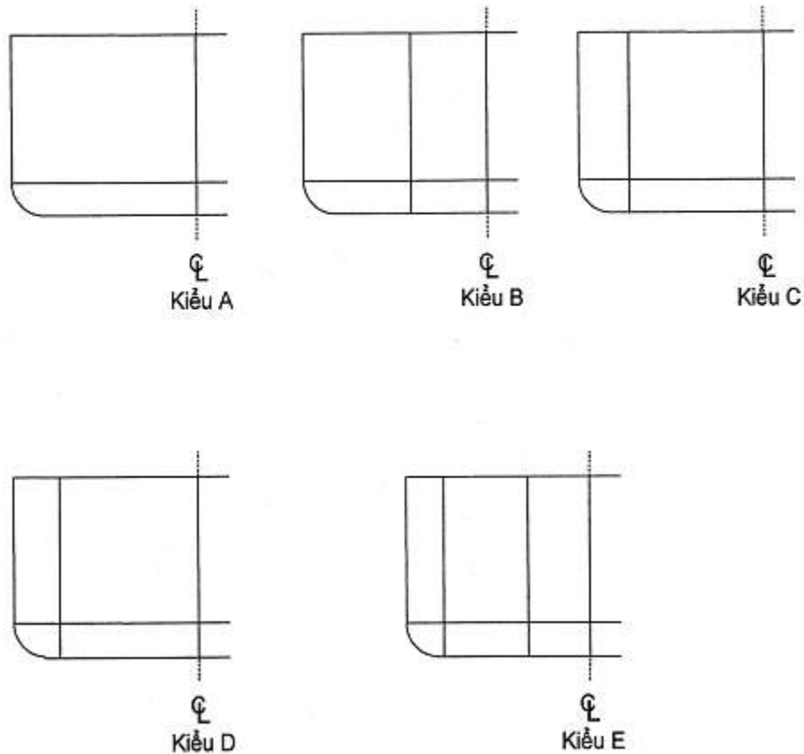
Hình 2A/13.6 Các kiểu tàu có vách dọc
