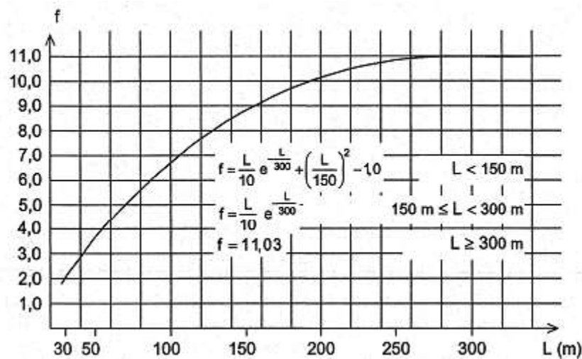
Hình 2A/8.1 Trị số của f
