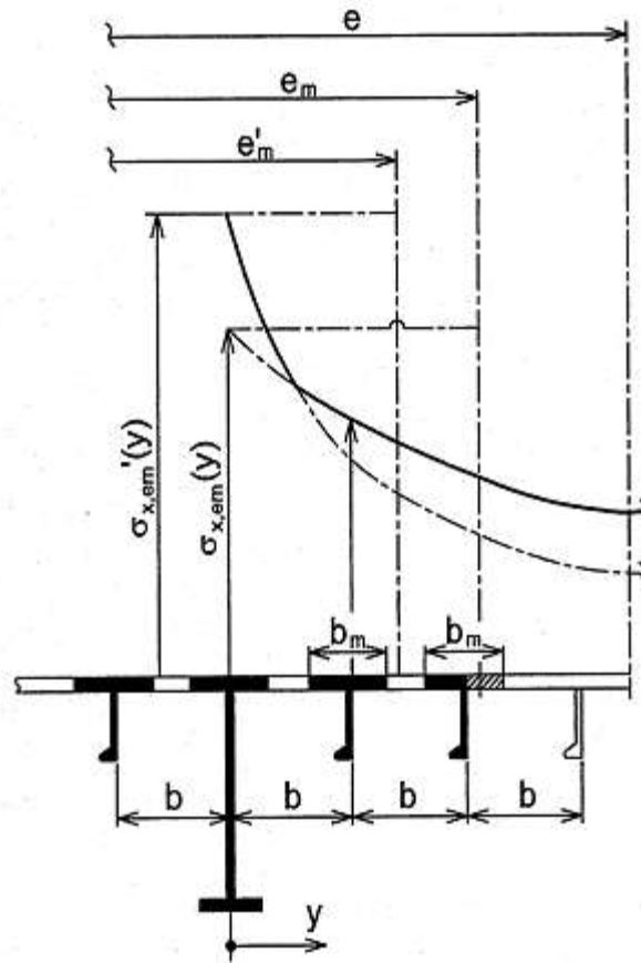
Hình 17.5 Nẹp đặt song song với bản thành của cơ cấu đỡ chính
