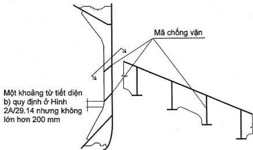
Hình 2A/29.16 Mã chống vắn
