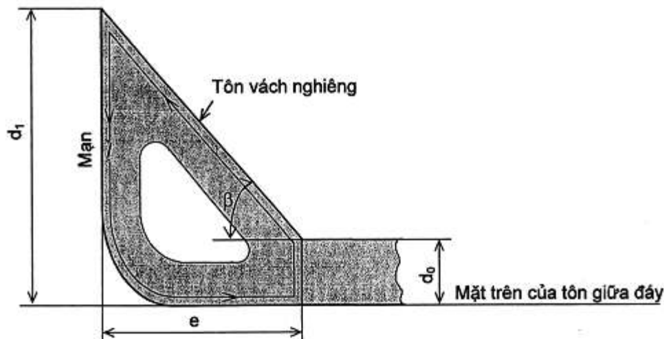
Hình 2A/29.1 Xác định \beta , l , e , d_0 , d_1
