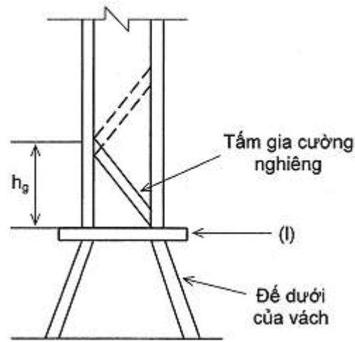
Hình 2A/29.7b Tấm gia cường nghiêng
