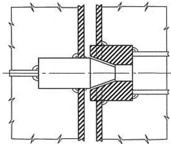
Hình 2A/21.4 Ví dụ về ổ chặn
