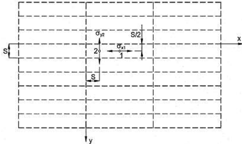
Hình 17.2 Xác định ứng suất pháp trên tấm nắp miệng khoang
