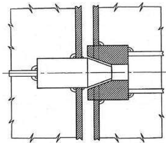
Hình 2B/19.4 Ví dụ về ổ chặn
