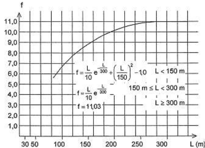
Hình 2A/16.1 Trị số của f
