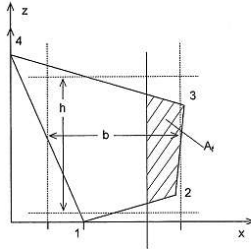
Hình 2A/25.2 Hệ thống tọa độ của bánh lái
