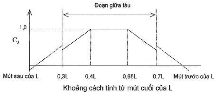
Hình 2B/13.1 Trị số của hệ số C_2
