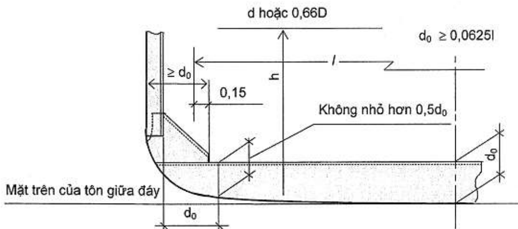
Hình 2A/3.1 Hình dạng của đà ngang đáy
