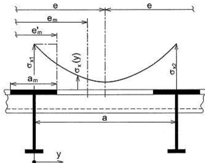
Hình 17.6 Nẹp đặt vuông góc với bản thành của cơ cấu đỡ chính
