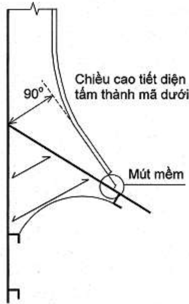
Hình 2A/29.15 Xác định chiều cao tiết diện tấm thành mã dưới khi tính t_{REN, dft}
