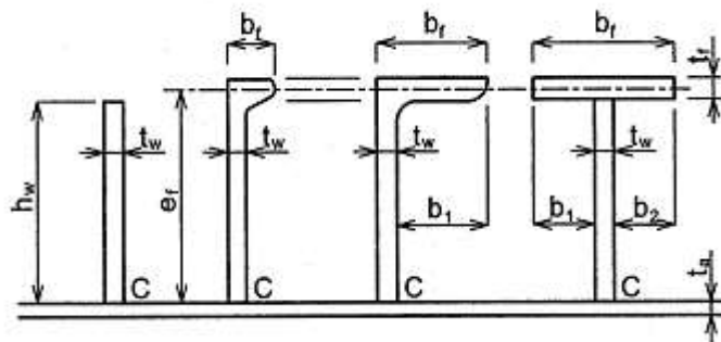
Hình 17.7 Các kích thước của nẹp
