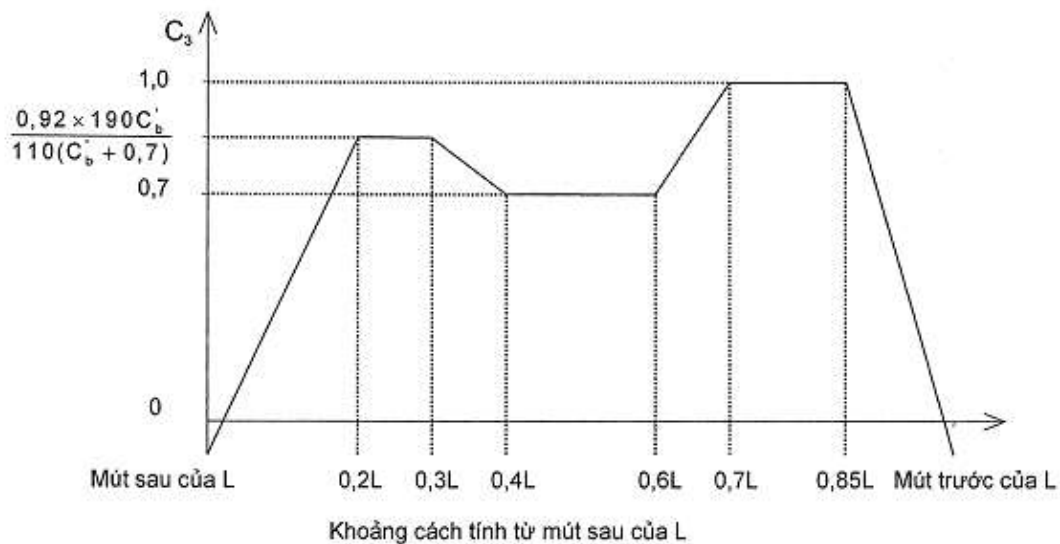
Hình 2A/13.4 Trị số của hệ số C_3
