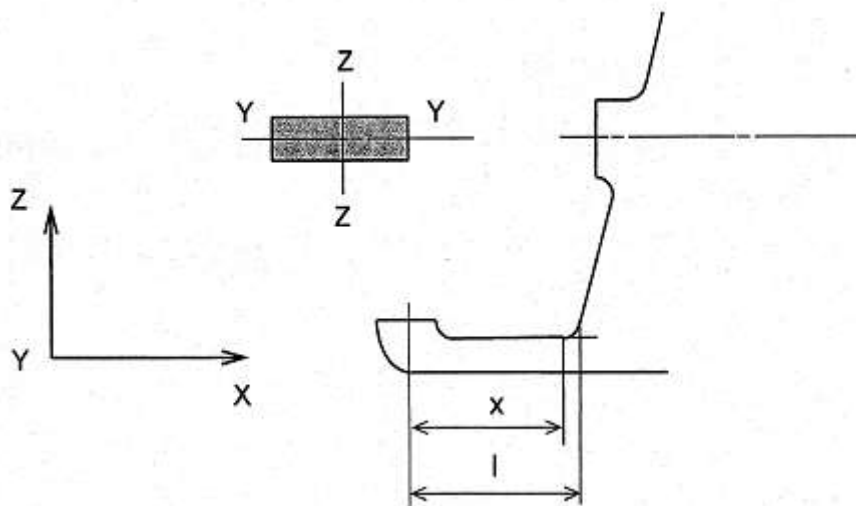
Hình 2A/2.2 Ky sóng đuôi
