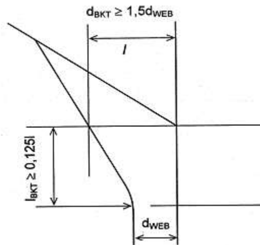
Hình 2A/29.4 Kích thước của mã nút
