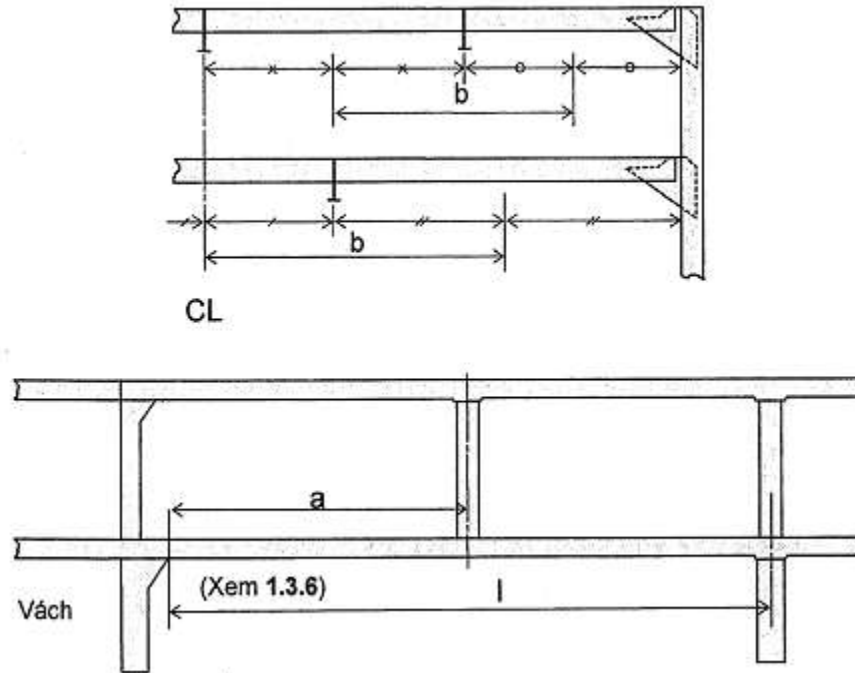
Hình 2B/10.1 Đo l, a và b
