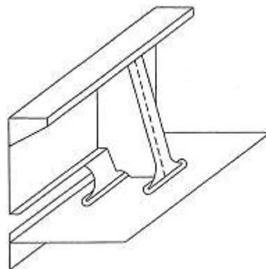
Hình 2A/21.2 Kiểu có tấm đệm
