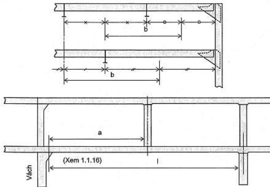
Hình 2A/10.1 Đo l, b và a
