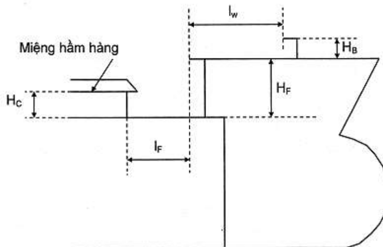
Hình 2A/16.2 Vị trí đặt thượng tầng mũi
