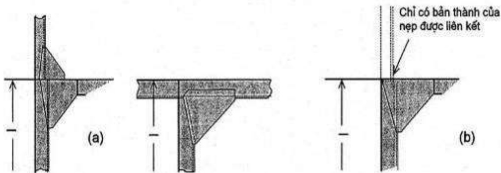
Hình 2A/11.1 Các kiểu liên kết nút
