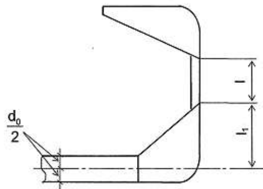
Hình 2A/29.2 Xác định l, l 1
