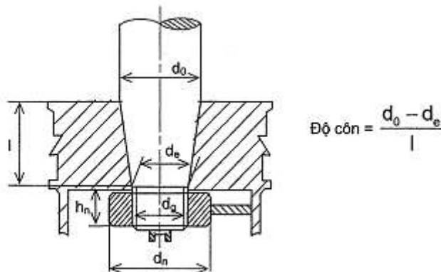
Hình 2A/25.4 Mỗi nối côn
