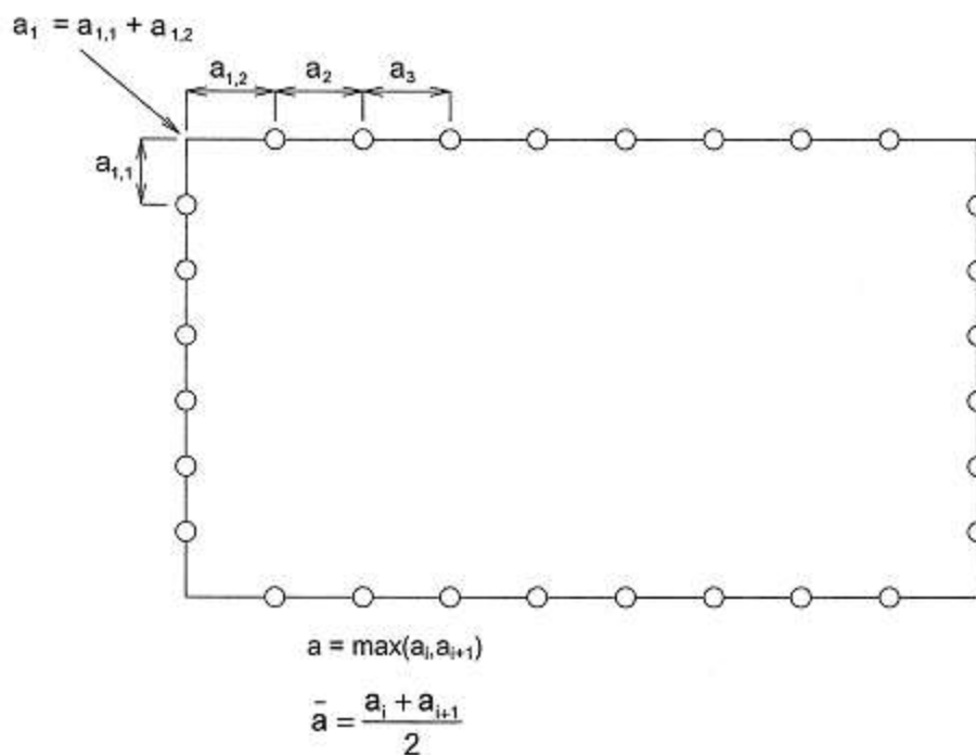
Hình 2A/18.3 Khoảng cách giữa các thiết bị cố định, đo dọc theo chu vi nắp miệng khoang
