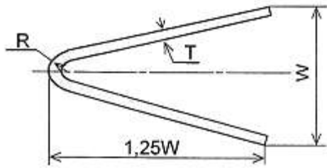
Hình 2A/2.1 Kích thước tiêu chuẩn của trụ chân vịt
