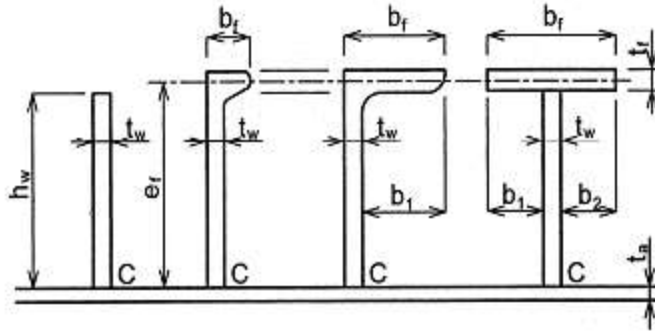
Hình 2A/18.7 Các kích thước của nẹp
