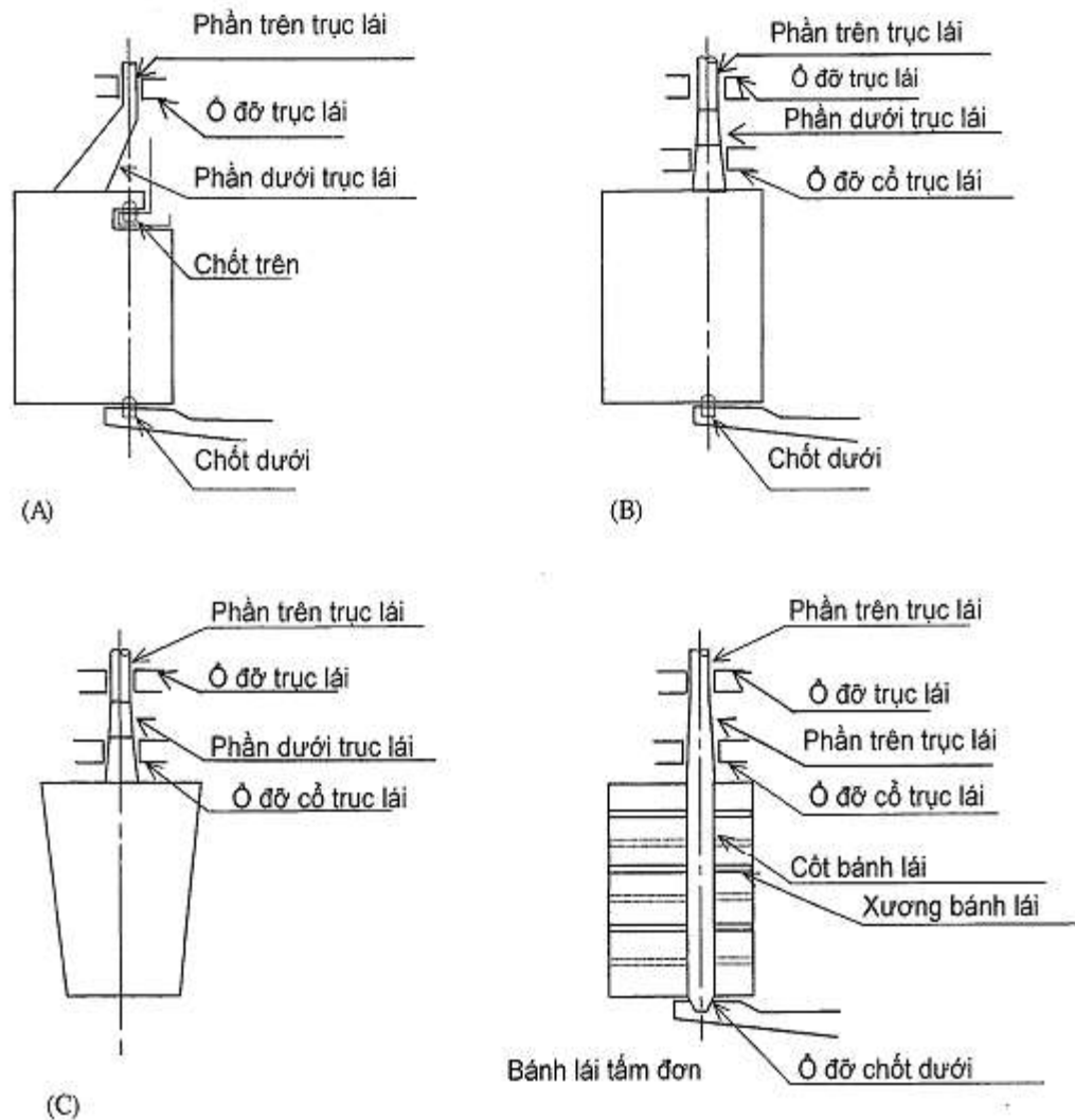
Hình 2B/21.1.1 Các dạng bánh lái
