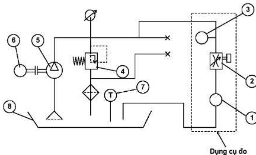
Hình 1 - Sơ đồ thử bơm
