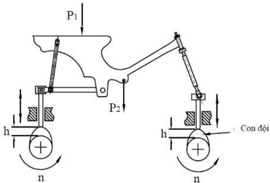
Hình 3. Sơ đồ nguyên lý kiểm tra độ bền khung xe với tải trọng động (Phương pháp 2)
