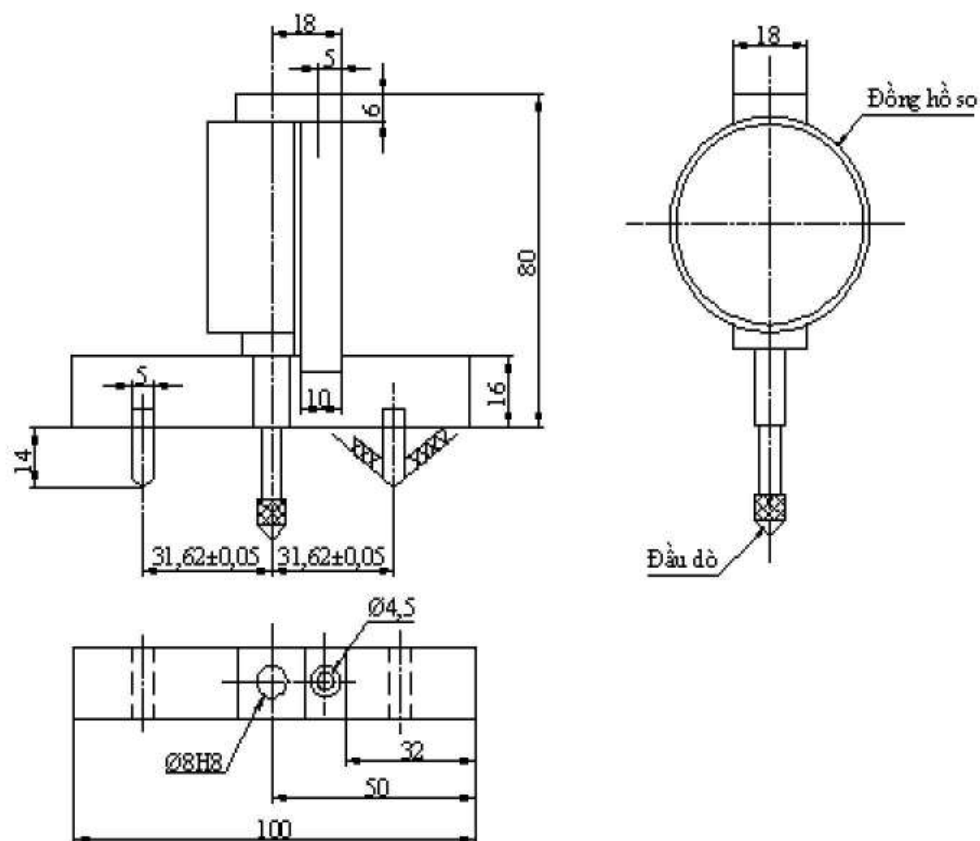
Hình B.1. Sơ đồ khái quát thiết bị đo bán kính cong
