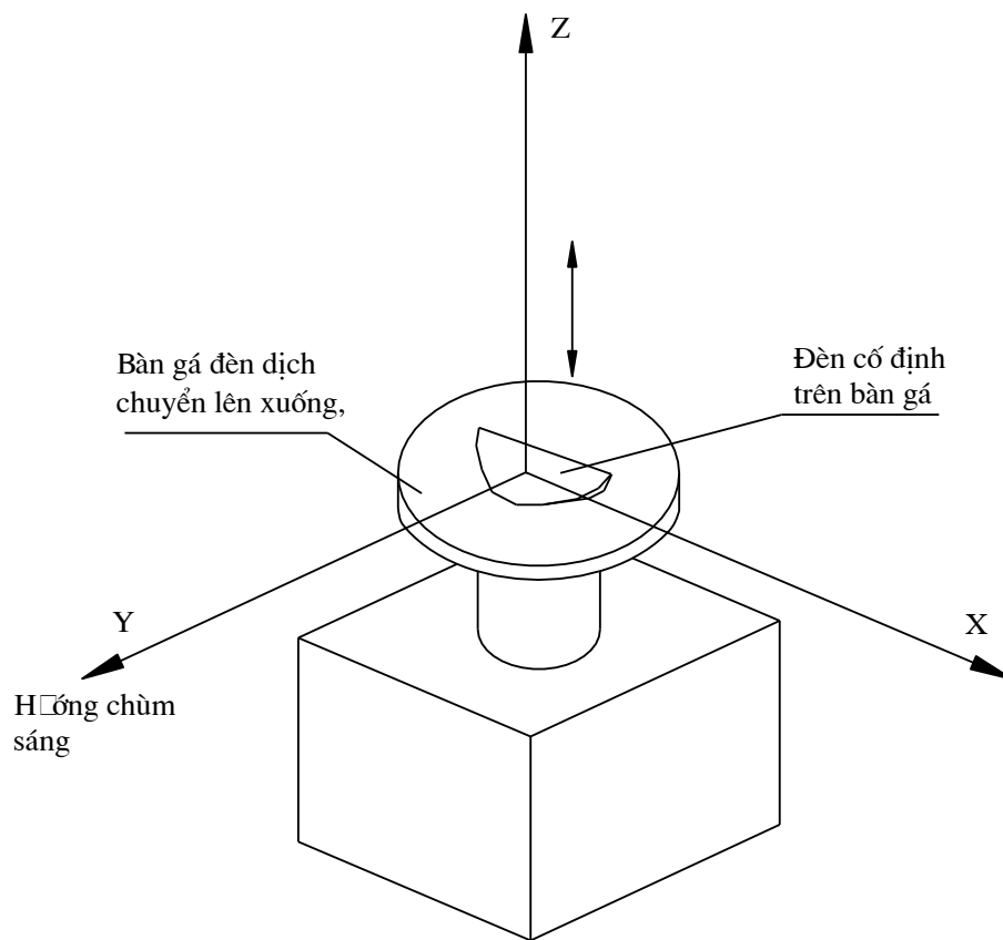
Hình 3: Bàn gá đèn theo nguyên lý 1.
