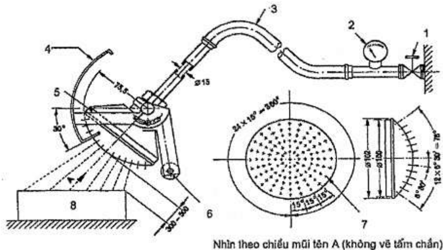
Hình 1. Thiết bị thử nghiệm về bảo vệ chống tia nước
