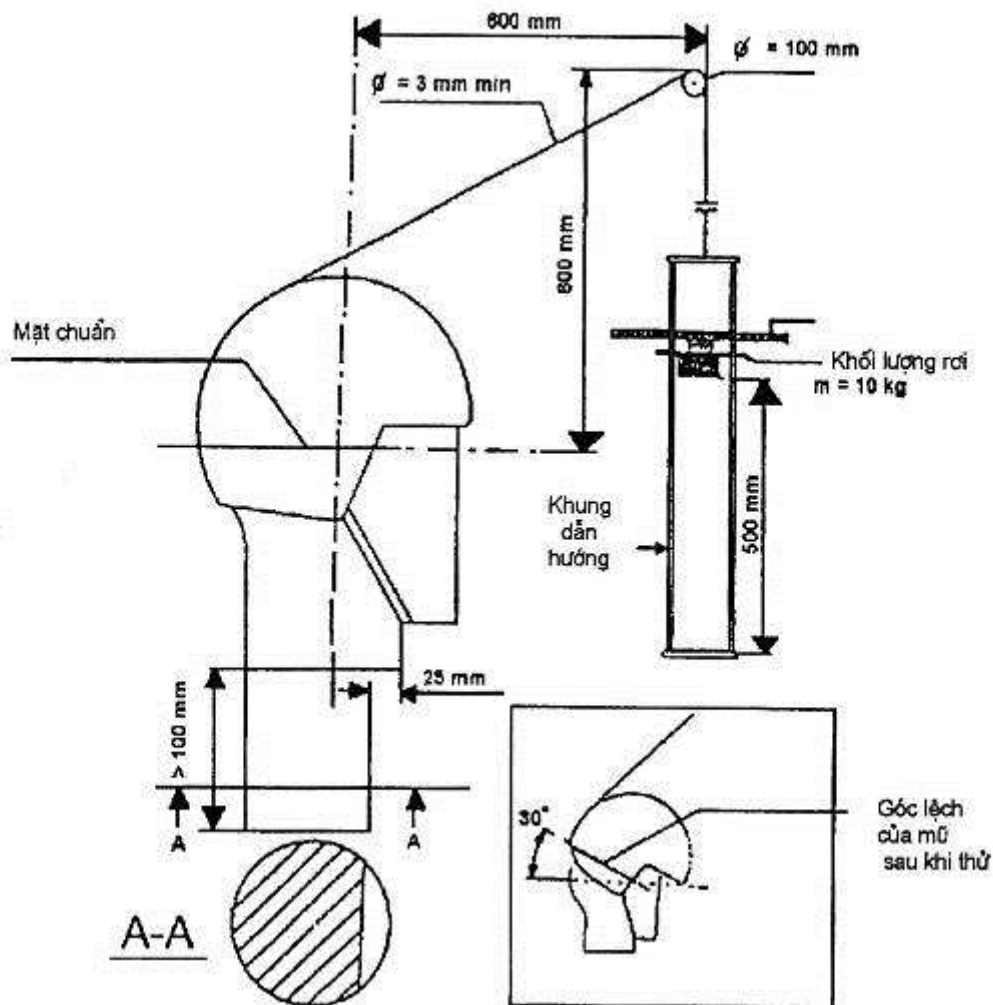
Hình 6 - Sơ đồ nguyên lý thử độ ổn định mũ
