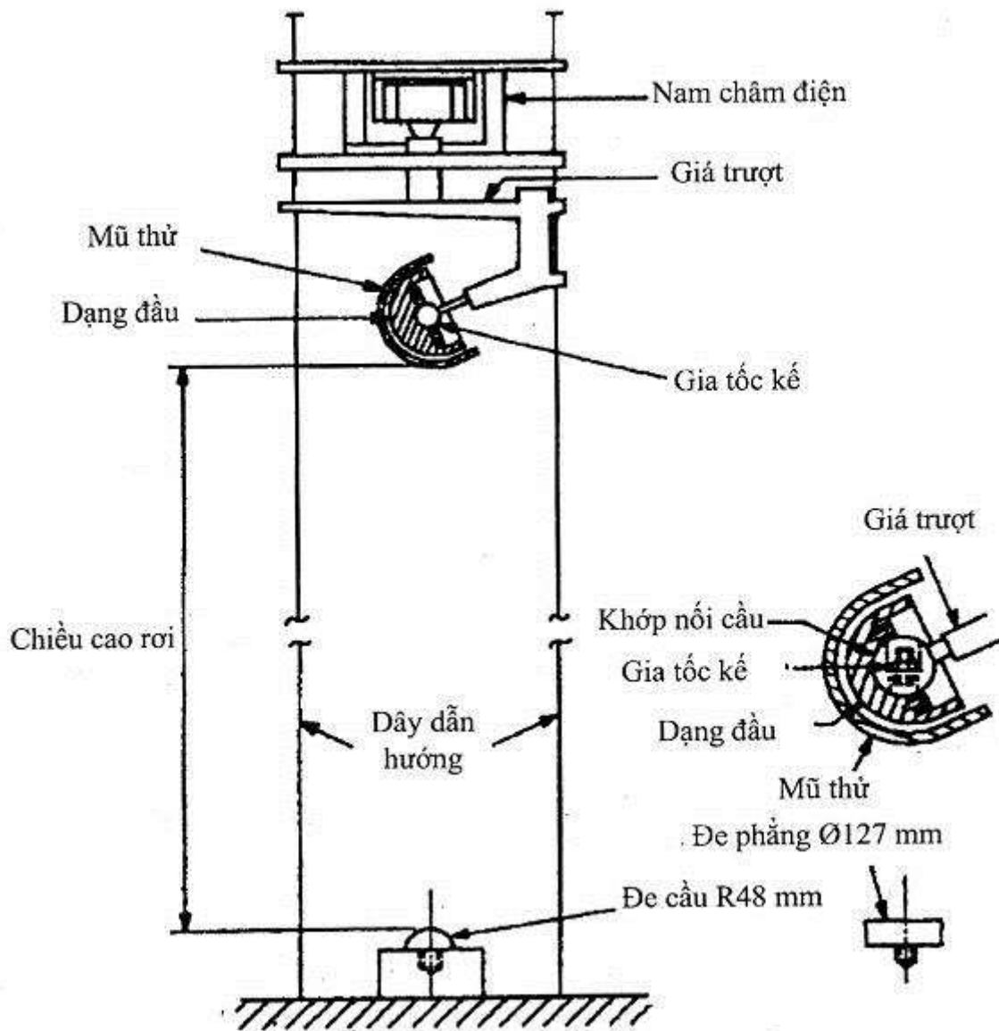
Hình3 - Sơ đồ nguyên lý thử độ bền va đập và hấp thụ xung động
